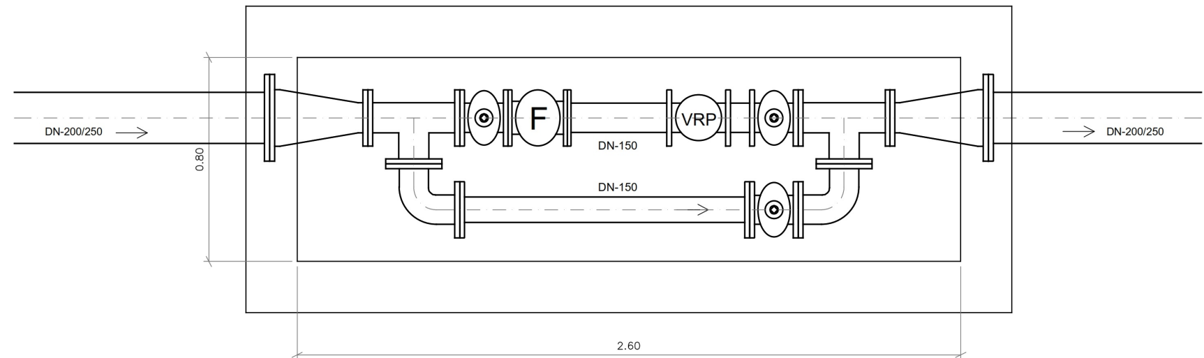
DETALL TIPUS B ARQUETA AMB REDUCTORA DE PRESSIÓ DN-150
