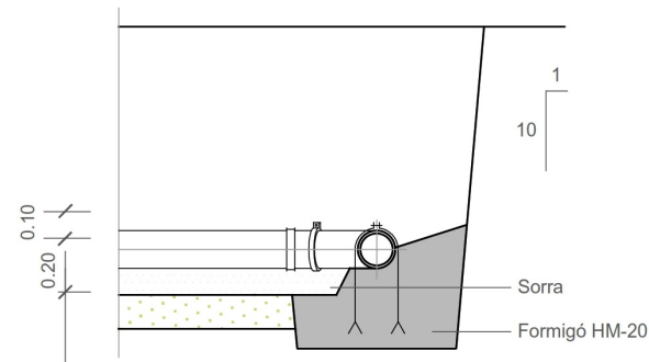
ANCORATGE Peces especials
