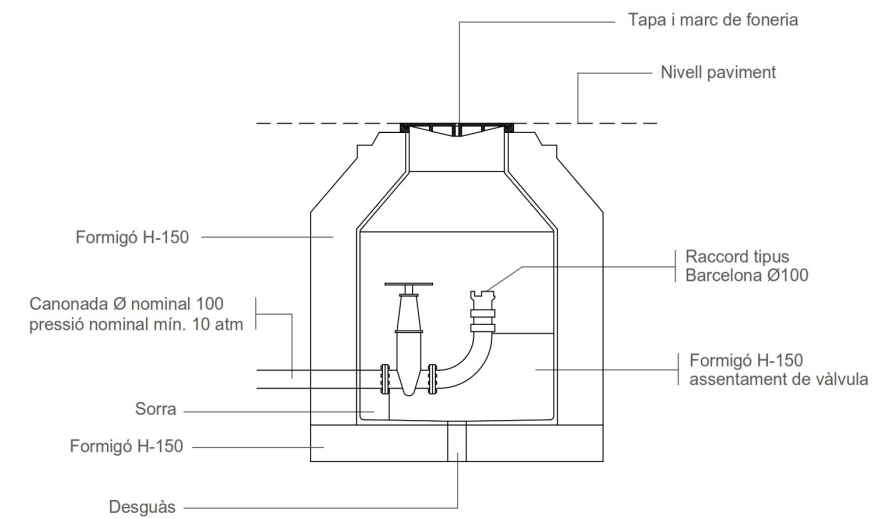
ALÇAT Troneta per a presa d'aigua per a hidrant
