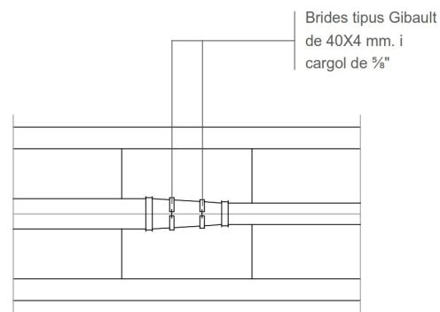
PLANTA CON DE REDUCCIÓ Peces especials
