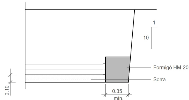
ALÇAT Peces especials
