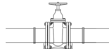
ALÇAT Detall vàlvula de seccionament
