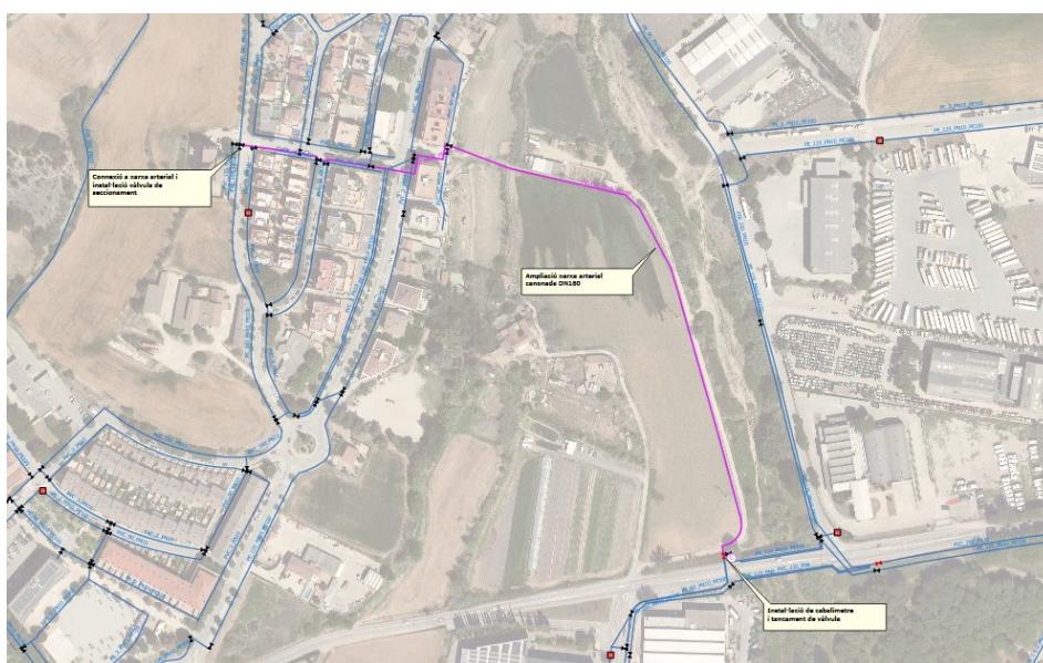
Imatge 17. Canonada arterial bypass els Batzacs DN 200 mm
