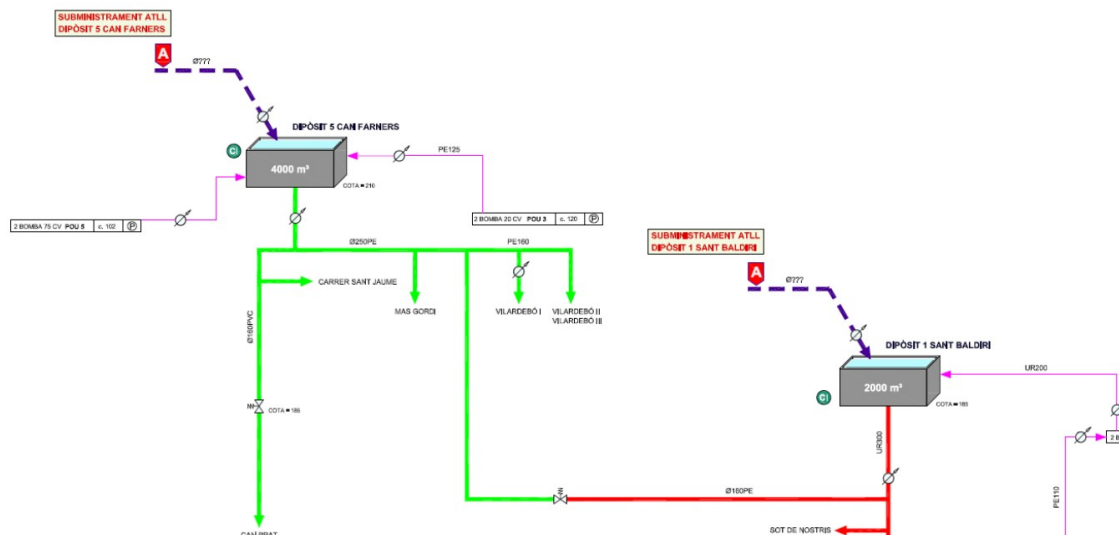
Figura 1. Esquema vertical xarxa en alta de Lliçà de Vall
