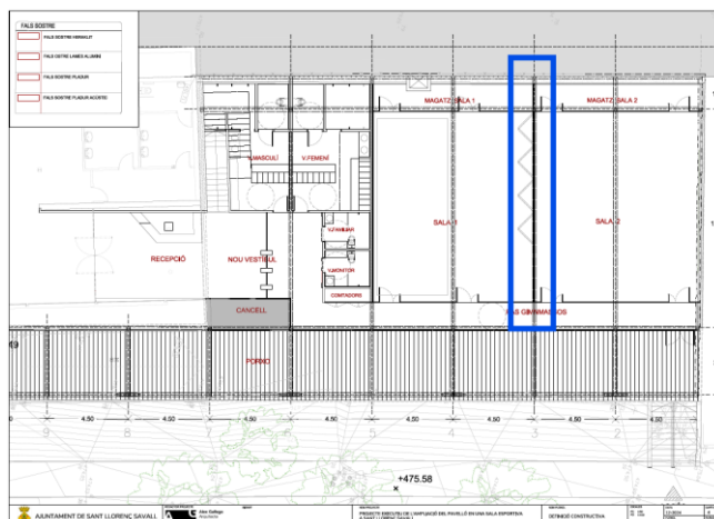
Retall sense escala plànol número 07 - planta baixa indicant ubicació envà mòbil
