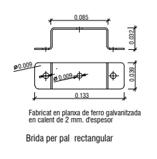
Detall constructiu. Peces d'ancoratge
