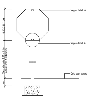
(* ) La part més desfavorable del senyal anirà retranquejada 60 cm. del cantó exterior de la vorera o voravia dels vials Detall constructiu. Senyal octogonal
