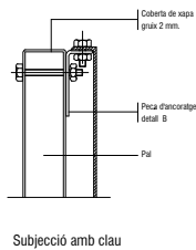
Subjecció amb clau
