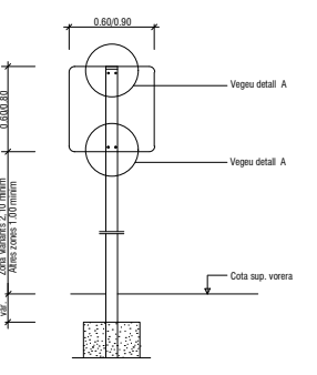
(* ) La part més desfavorable del senyal anirà retranquejada 60 cm. del cantó exterior de la vorera o voravia dels vials Detall constructiu. Senyal quadrada
