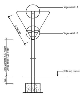
(* ) La part més desfavorable del senyal anirà retranquejada 60 cm. del cantó exterior de la vorera o voravia dels vials Detall constructiu. Senyal triangular invertida
