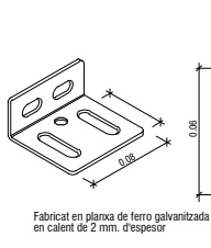
Fabricat en planxa de ferro galvanitzada en calent de 2 mm. d'espessor Brida per pal rodó
