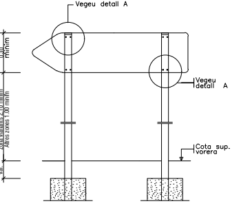
(* ) La part més desfavorable del senyal anirà retranquejada 60 cm. del cantó exterior de la vorera o voravia dels vials Detall constructiu. Senyal de direcció pròpia
