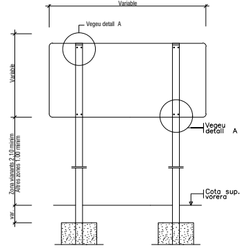
(* ) La part més desfavorable del senyal anirà retranquejada 60 cm. del cantó exterior de la vorera o voravia dels vials Detall constructiu. Senyal rectangular horitzontal
