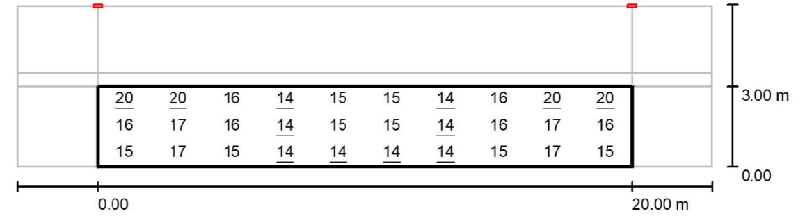
Valores en Lux, Escala 1 : 186
