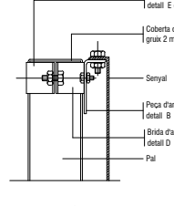
Subjecció amb brida
