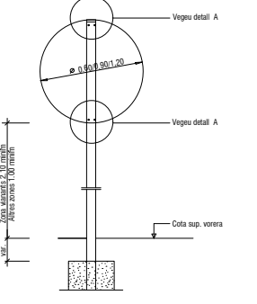
(* ) La part més desfavorable del senyal anirà retranquejada 60 cm. del cantó exterior de la vorera o voravia dels vials Detall constructiu. Senyal circular
