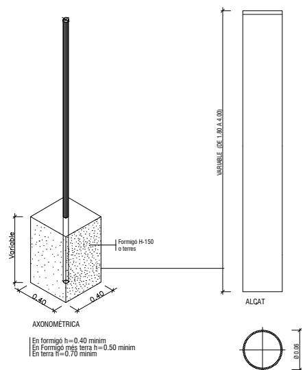
Pal de sustentament de senyals. Circulars GRUXX XAPA 2 mm. MINIM SECCIÓ
