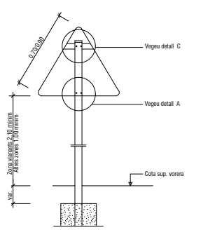
(* ) La part més desfavorable del senyal anirà retranquejada 60 cm. del cantó exterior de la vorera o voravia dels vials Detall constructiu. Senyal triangular
