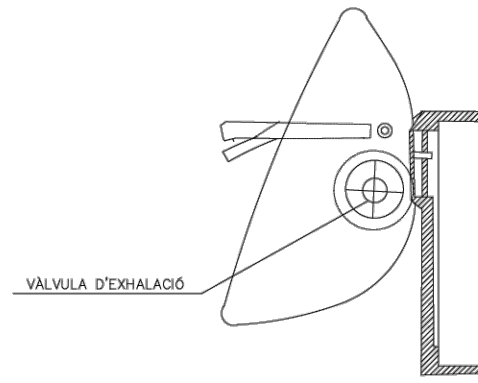
SECCIÓ A-A
