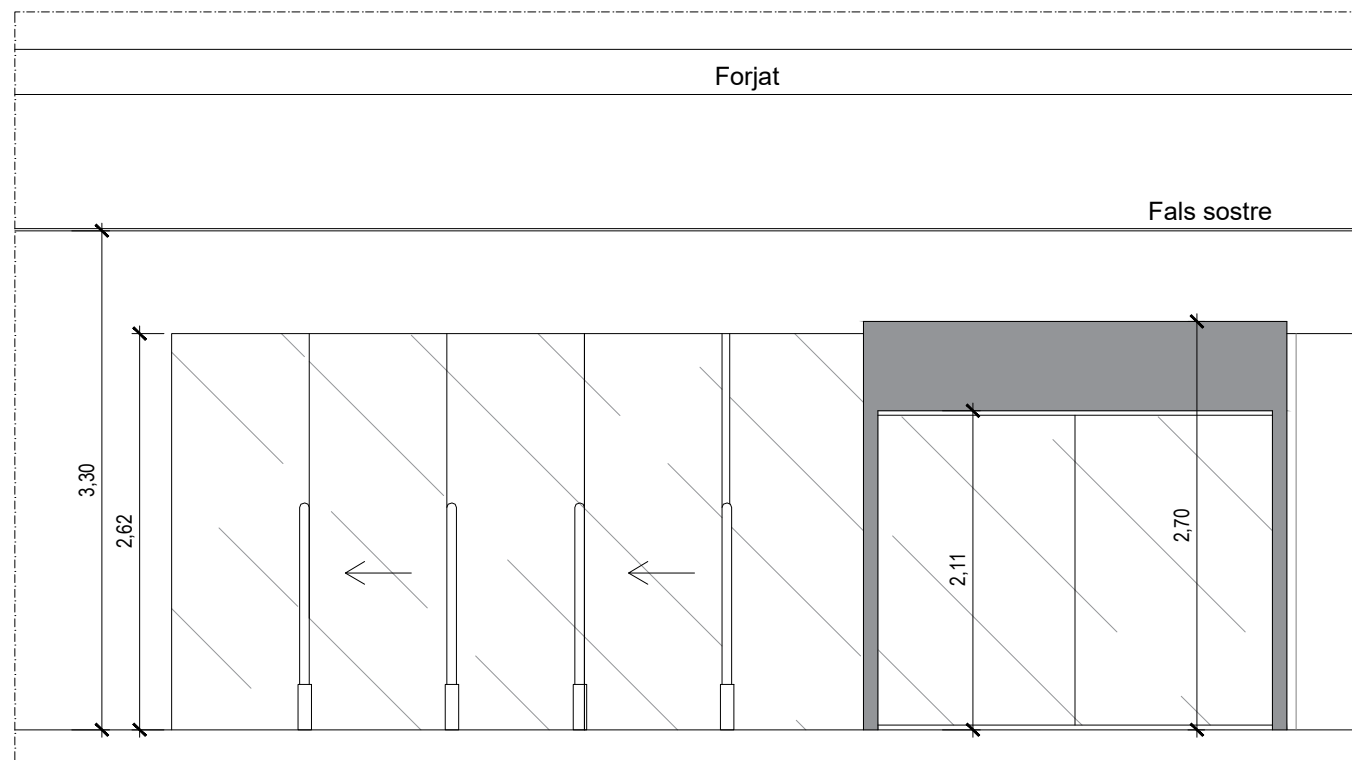
ESTAT ACTUAL DETALL ALÇAT FRONTAL e. 1/50
