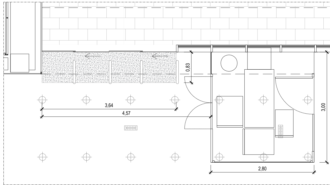
ESTAT ACTUAL DETALL PLANTA e. 1/50
