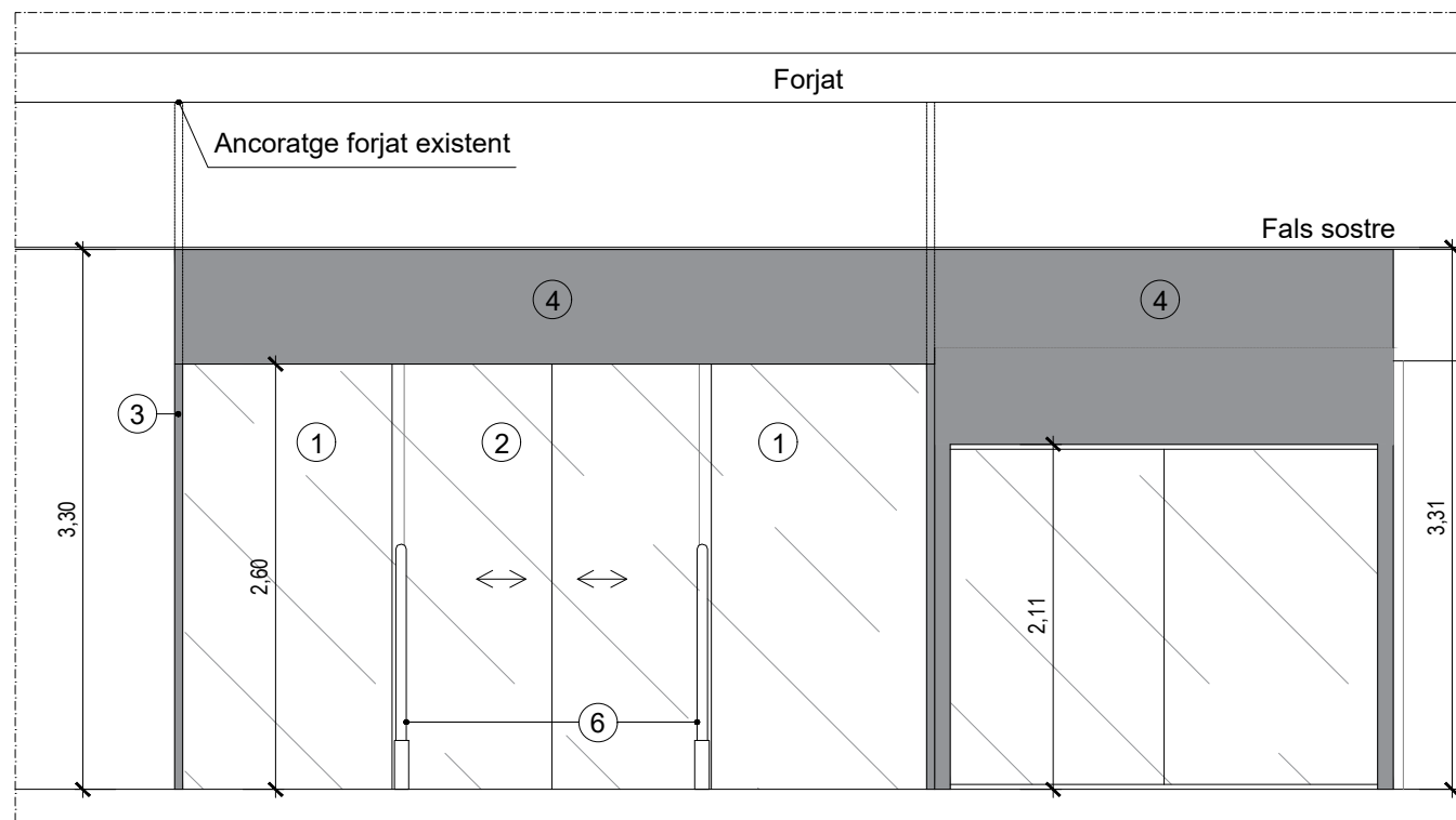
DETALL PROPOSTA ALÇAT FRONTAL e. 1/50
