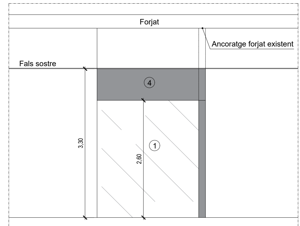
DETALL PROPOSTA ALÇAT LATERAL e. 1/50
