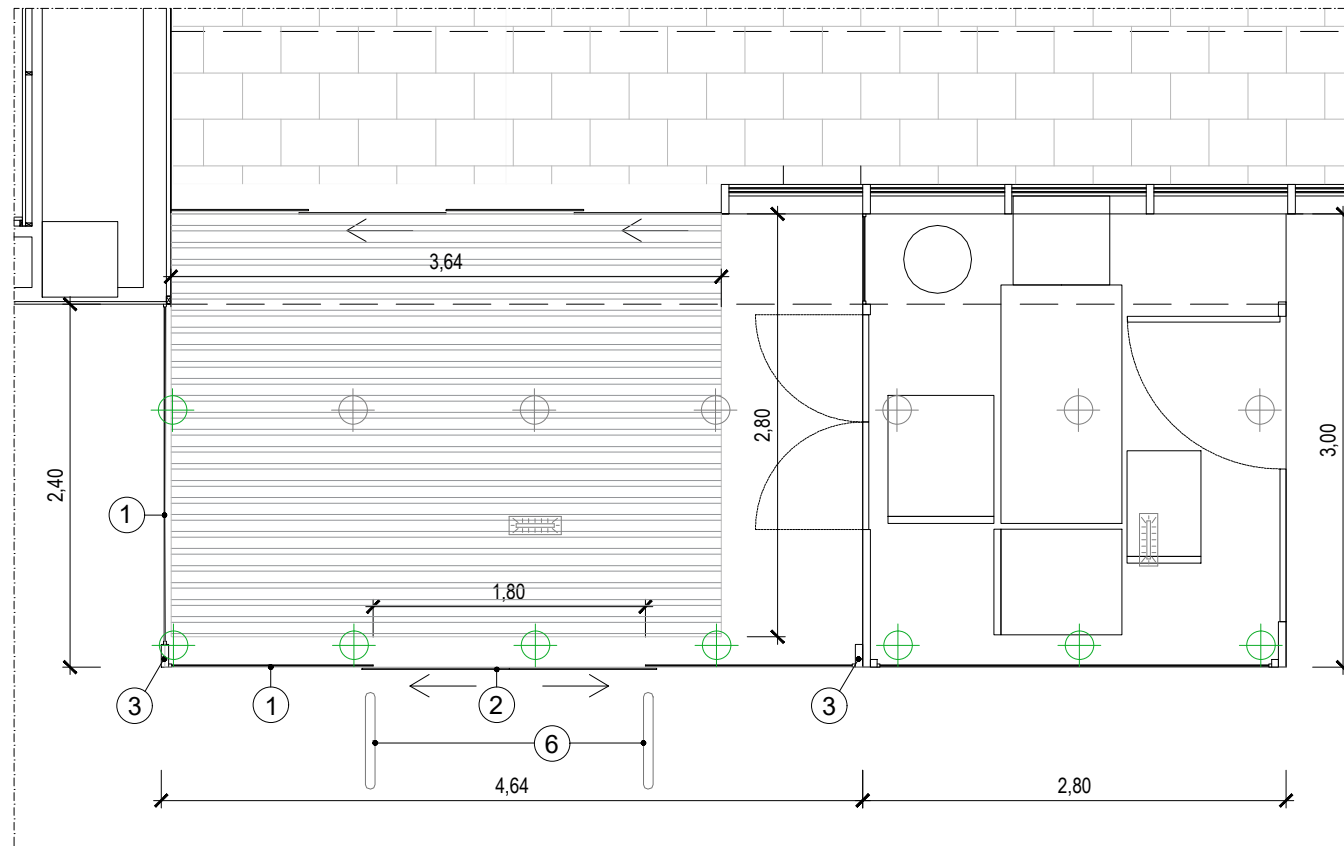
DETALL PROPOSTA PLANTA e. 1/50
