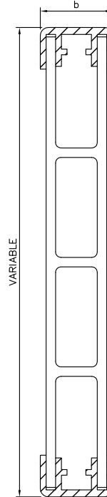
TIPUS "D"
