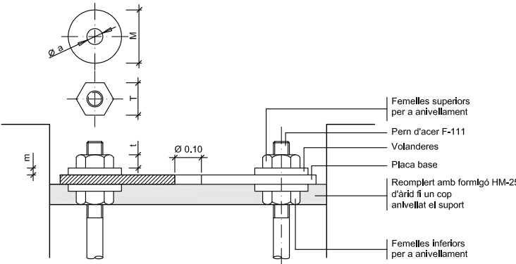
Detall ancoratges de les columnes i bàculs
