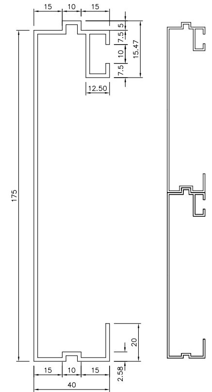
TIPUS "E"
