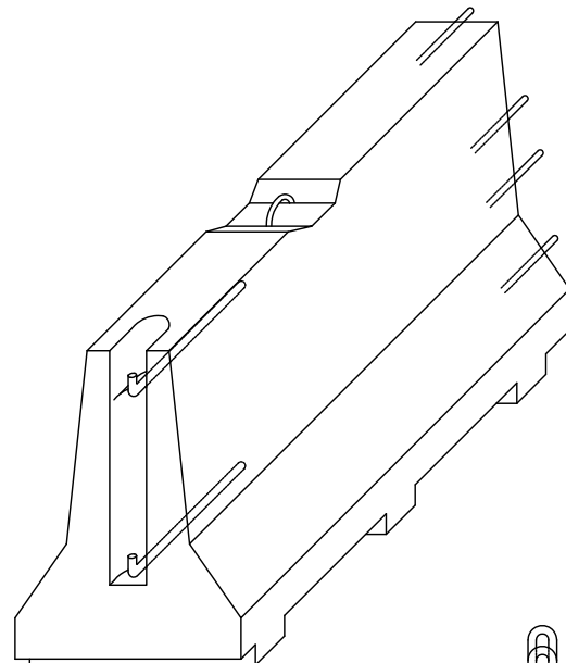
AXONOMÈTRICA
