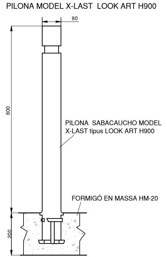
PILONA E: 1/10
