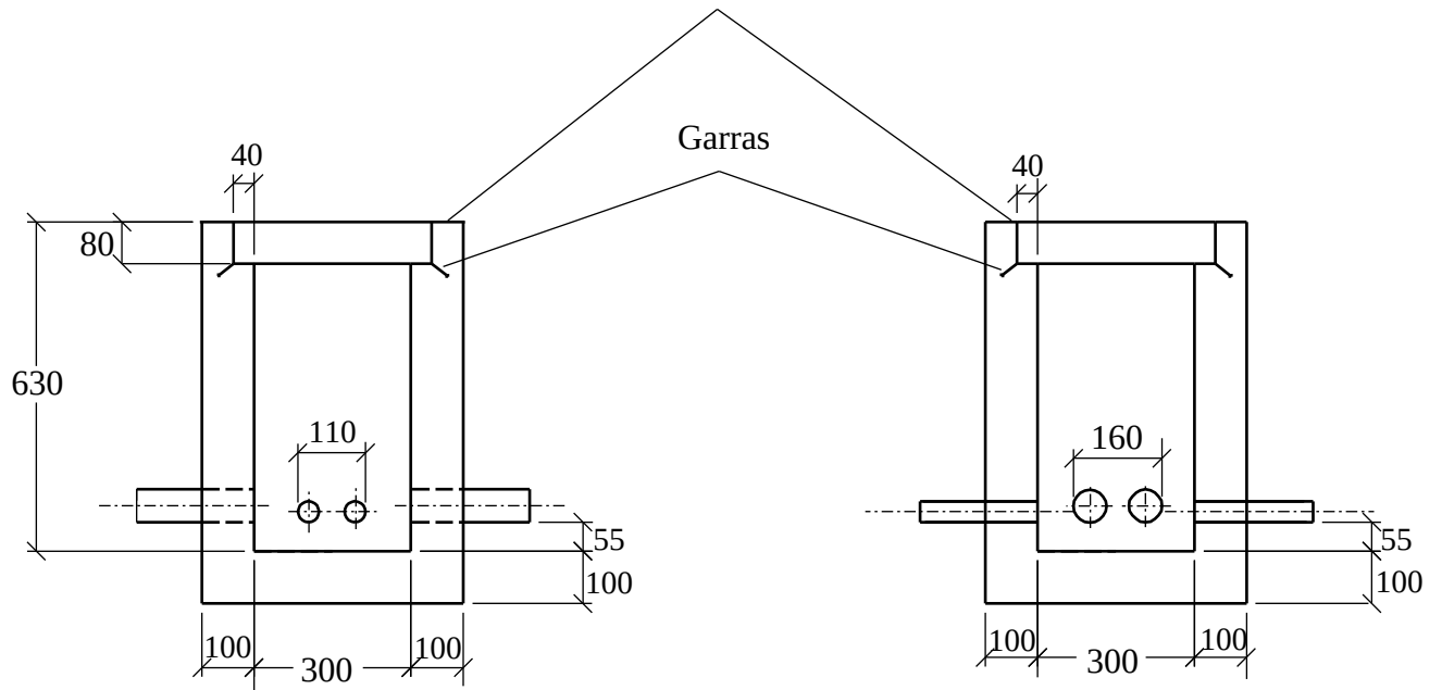
SECCIÓN A-A'
