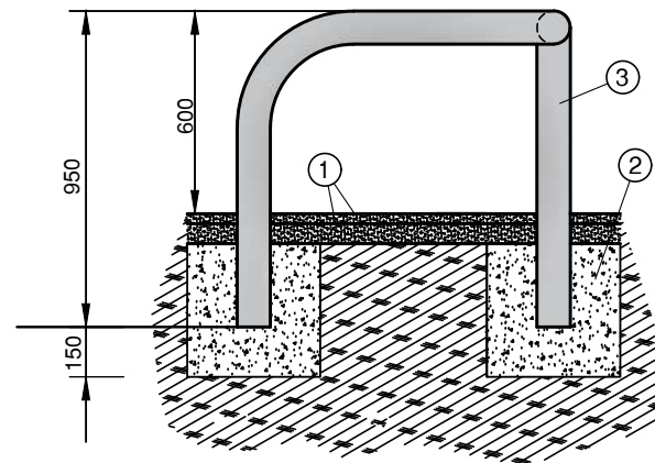
PROTECTOR APARCAMENT ALÇAT
