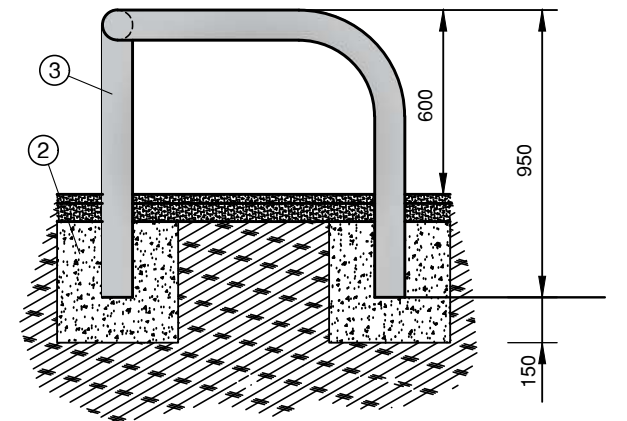
PROTECTOR APARCAMENT ALÇAT
