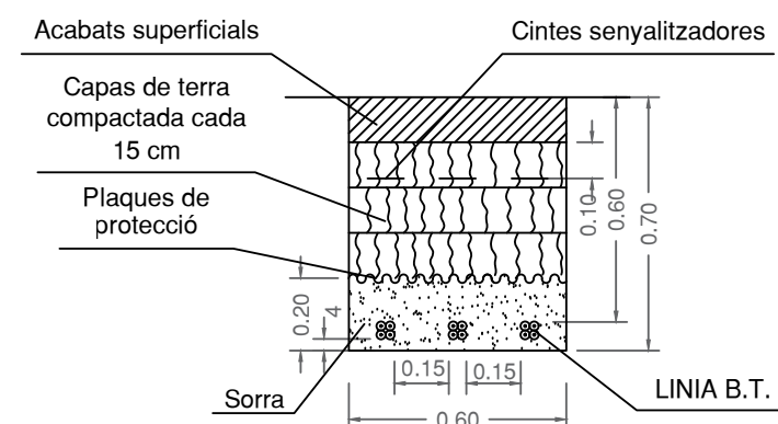
DETALL RASA TRES CIRCUITS
