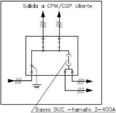
ESQUEMA UNIFILAR CAJA DE DISTRIBUCIÓN URBANA
