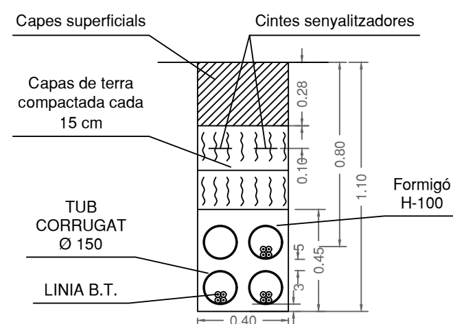
DETALL RASA TRES CIRCUITS
