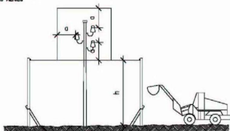
PÒRTIC DE BAIXAMENT PROTECCIÓ DE LÍNEES ELÈCTRIQUES AÈRIES
