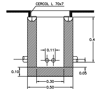
SECCIÓ A-A'
