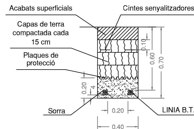
DETALL RASA DOS CIRCUITS
