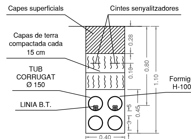
DETALL RASA DOS CIRCUITS
