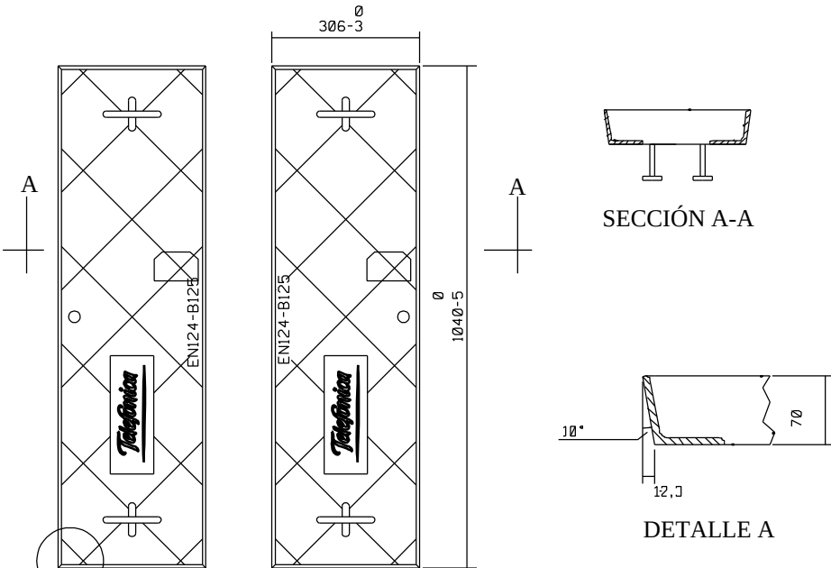
TAPA PREFABRICADA DE HORMIGÓN
