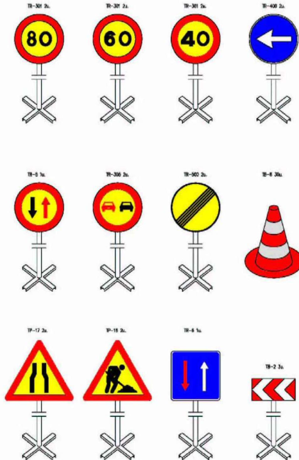
EQUIP ESTANDARD - SENYALITZACIÓ D'OBRES PER CARRETERA CONVENCIONAL - SENYALS AMB FONS GROC
