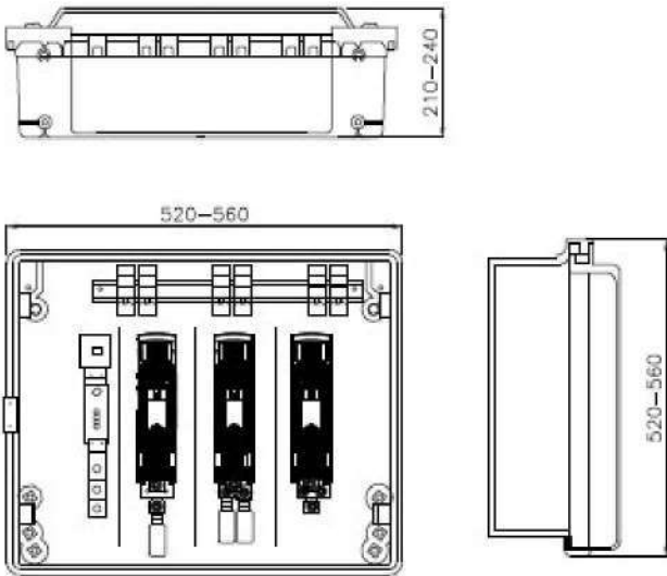
CAJA DISTRIBUCIÓN URBANA (CDU) s/norma informativa CNL004
