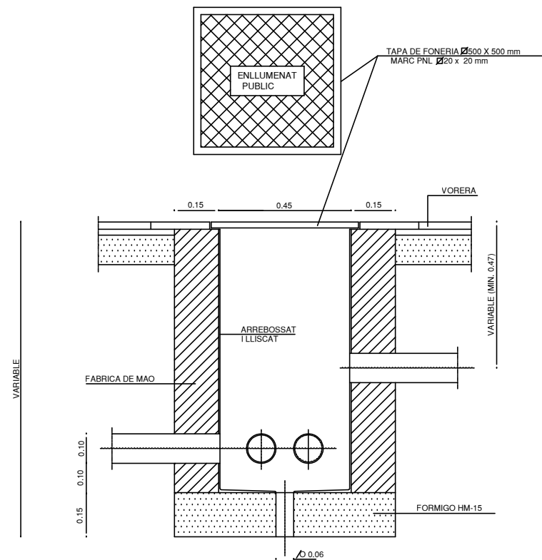
ARQUETA DE CONNEXIONS TIPUS
