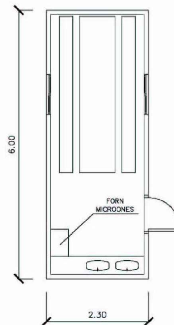
CASETA MOBIL PER A MENJADOR D'OBRA (10 PERSONES)
