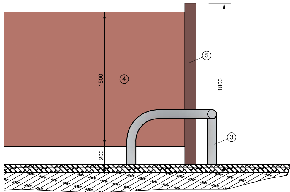
PROTECTOR CONTENIDORS ALÇAT
