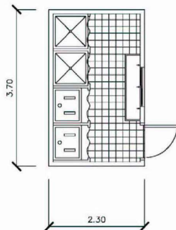
CASETA MOBIL PER A SERVEIS HIGIENICS D'OBRA
