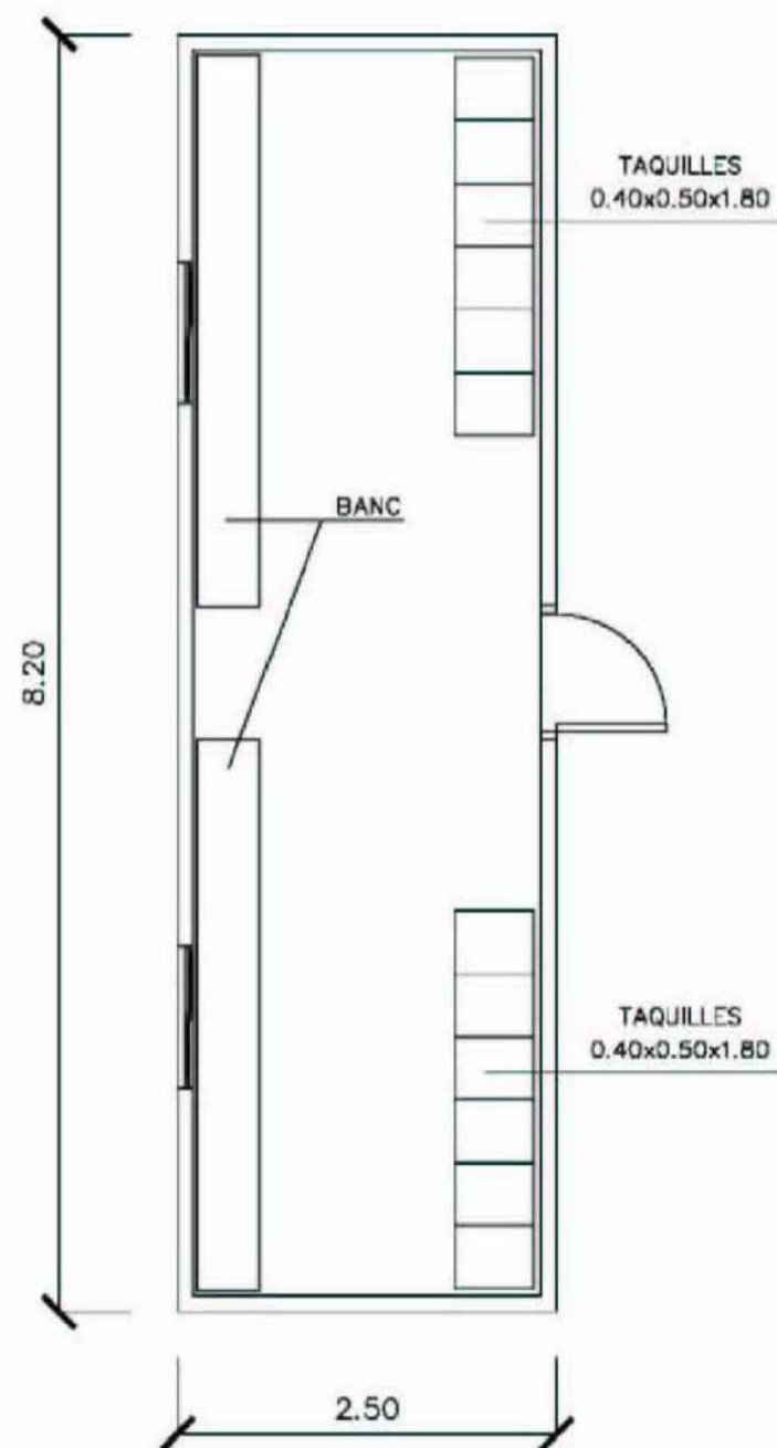
CASETA MOBIL PER A VESTIDORS D'OBRA
