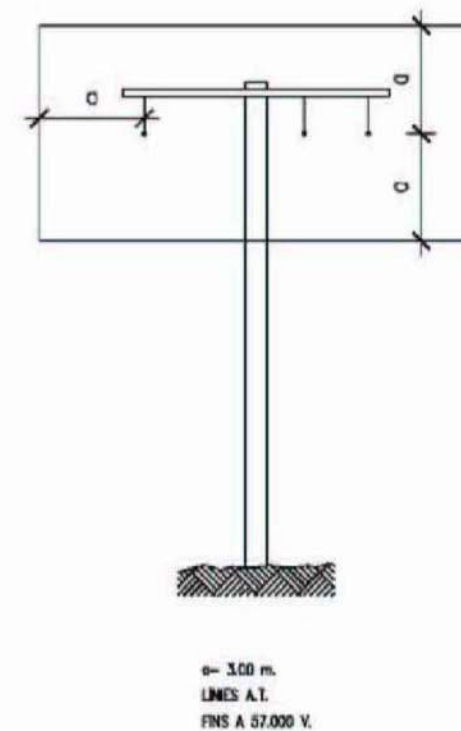
DISTÀNCIES RELATIVES DE PROTECCIÓ PER A MAQUINÀRIA D'OBRA PROPERA A LES LÍNEES ELÈCTRIQUES AÈRIES
