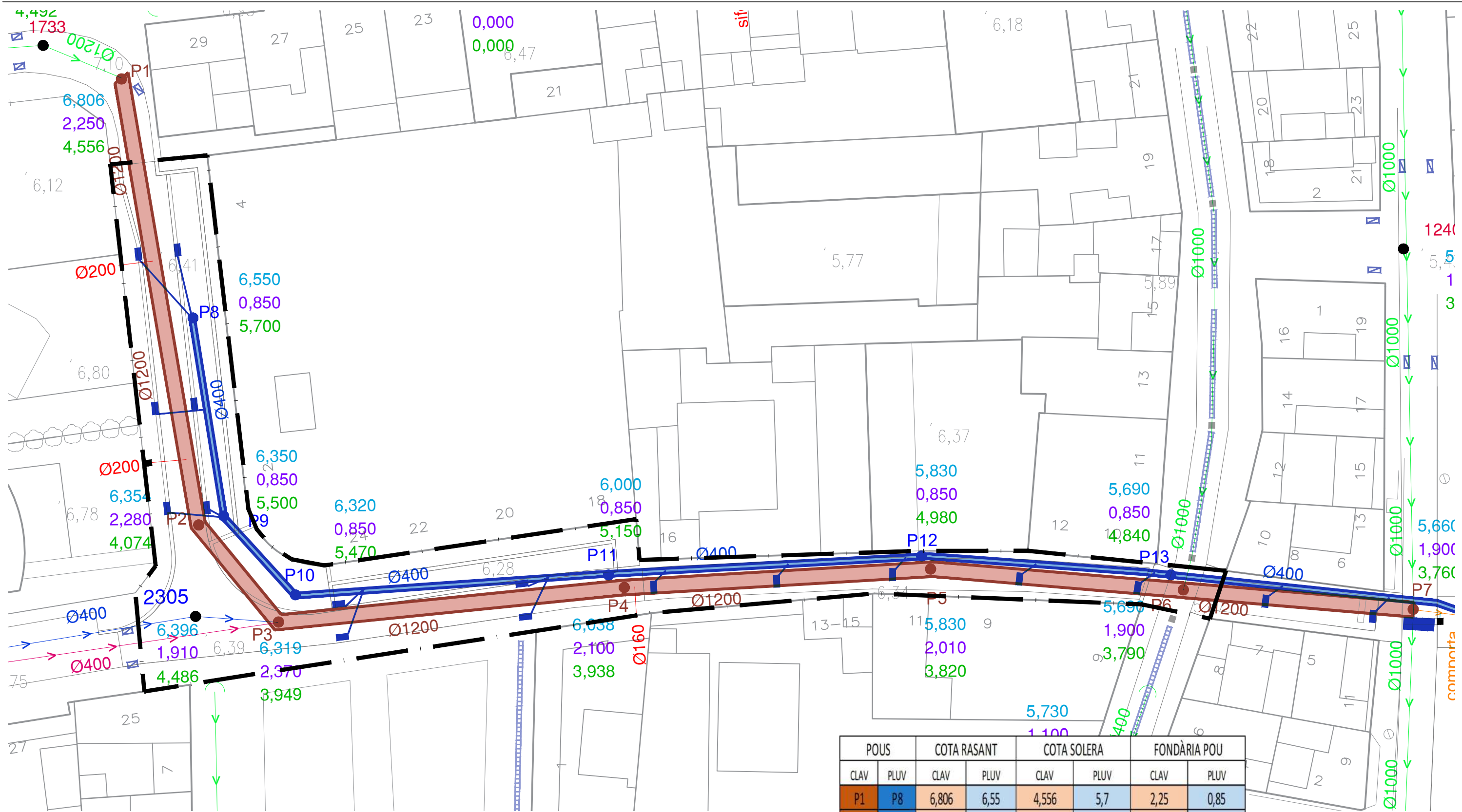
LLEGGENDA CLAVEGUERAM PROPOSTA
