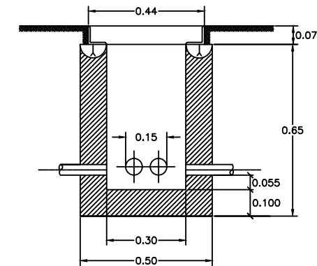
SECCIÓ B-B'
