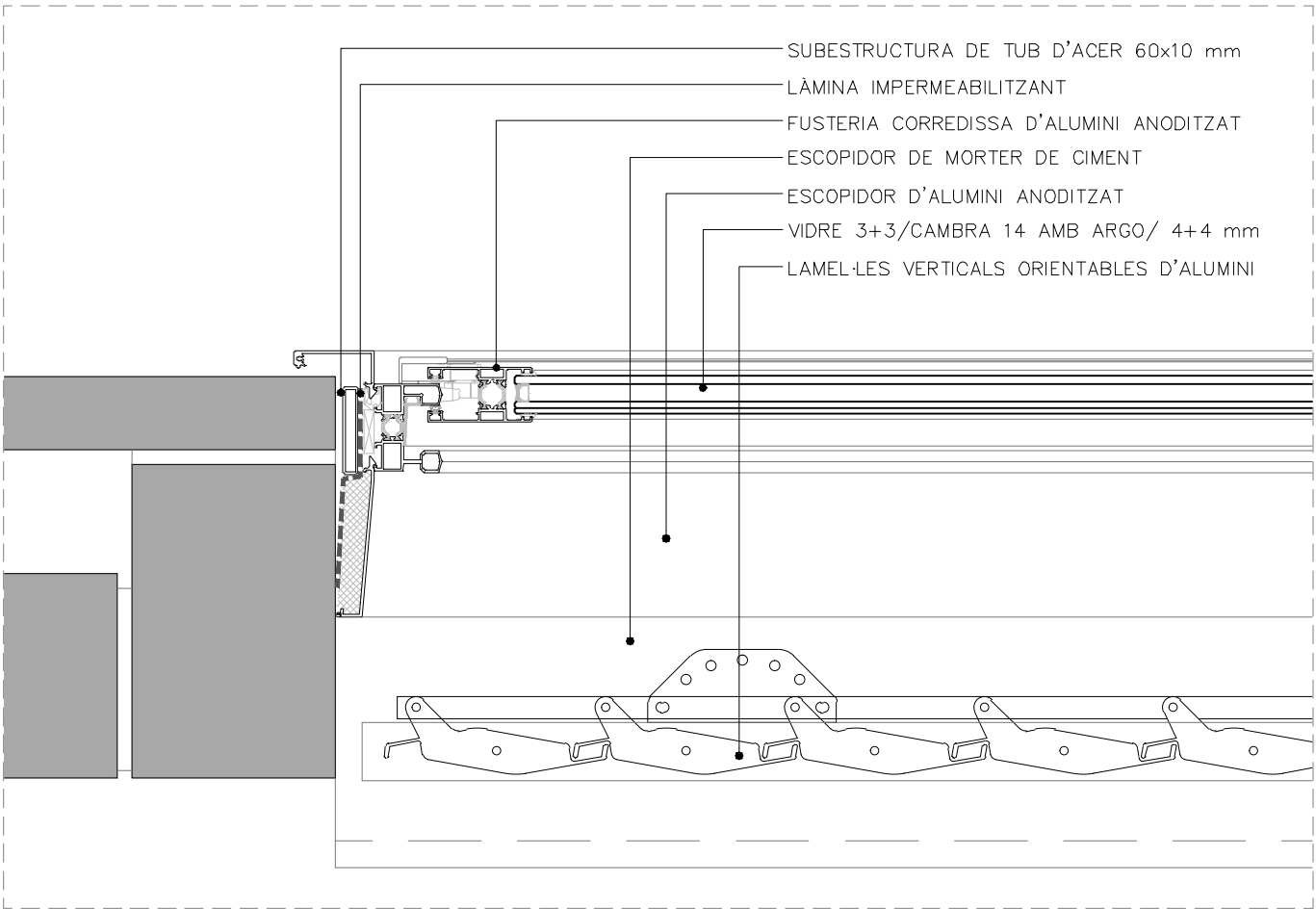
DETALL PLANTA 3
