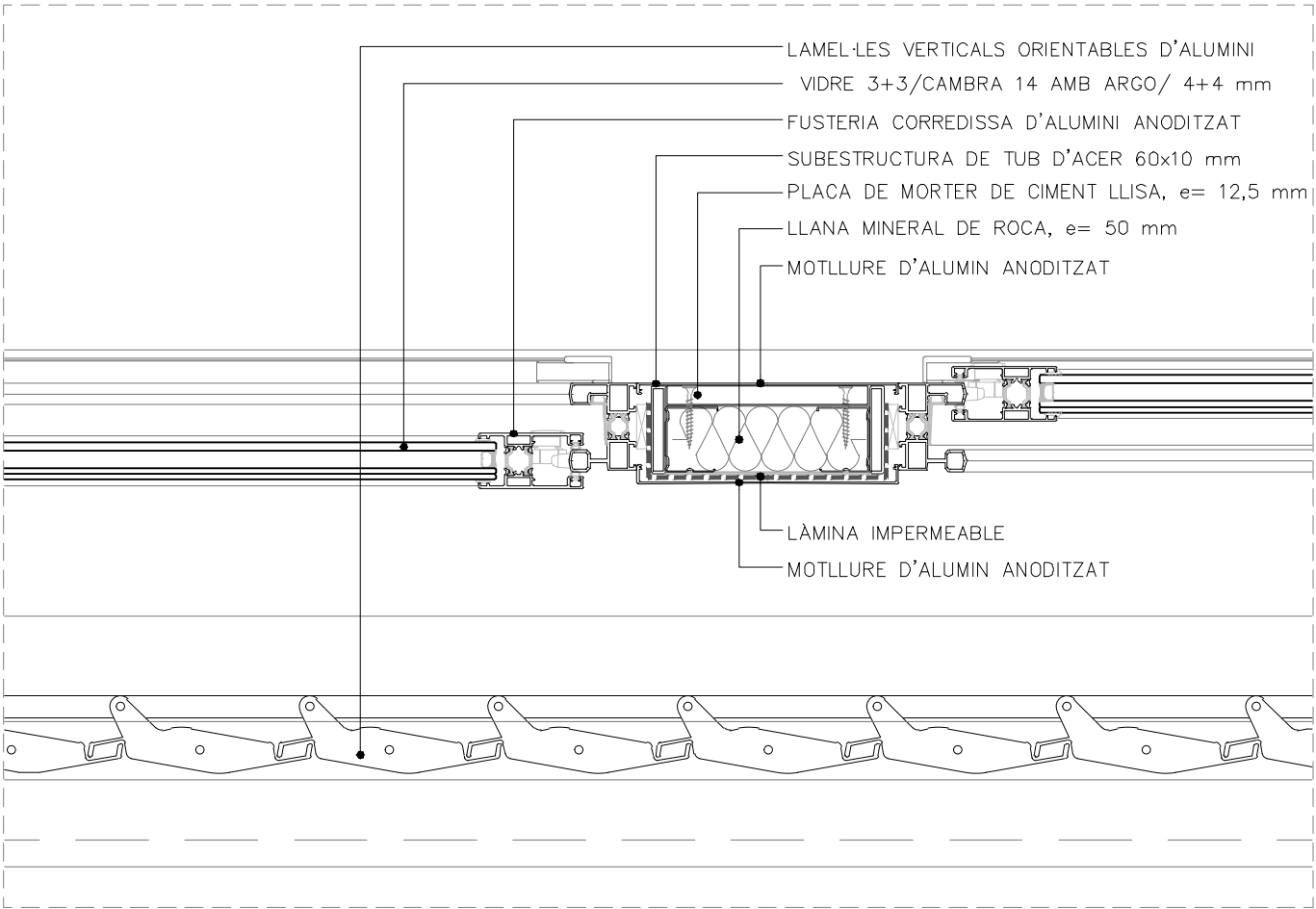
DETALL PLANTA 4
