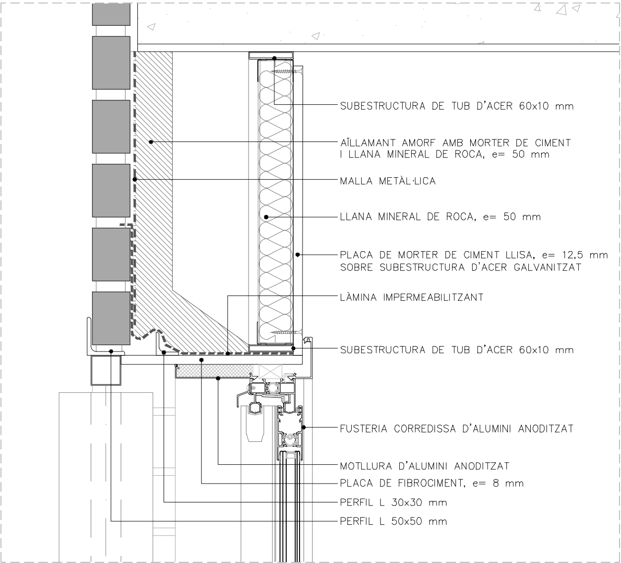
DETALL SECCIÓ 1
