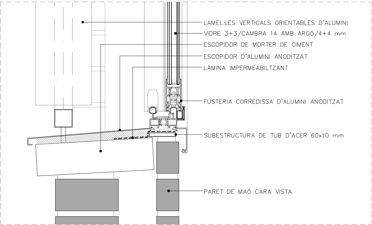
DETALL SECCIÓ 2
