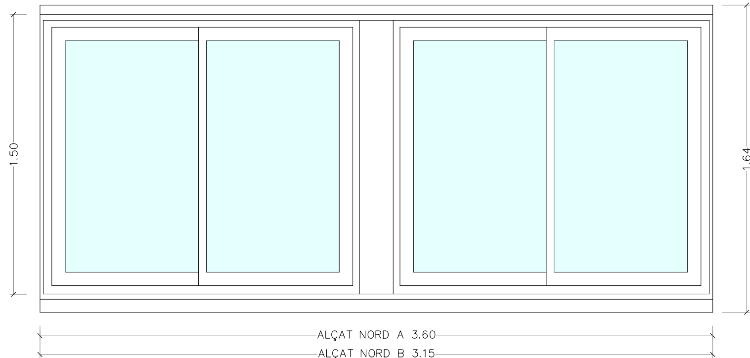
ALÇAT FINESTRA TIPUS. FUSTERIA
