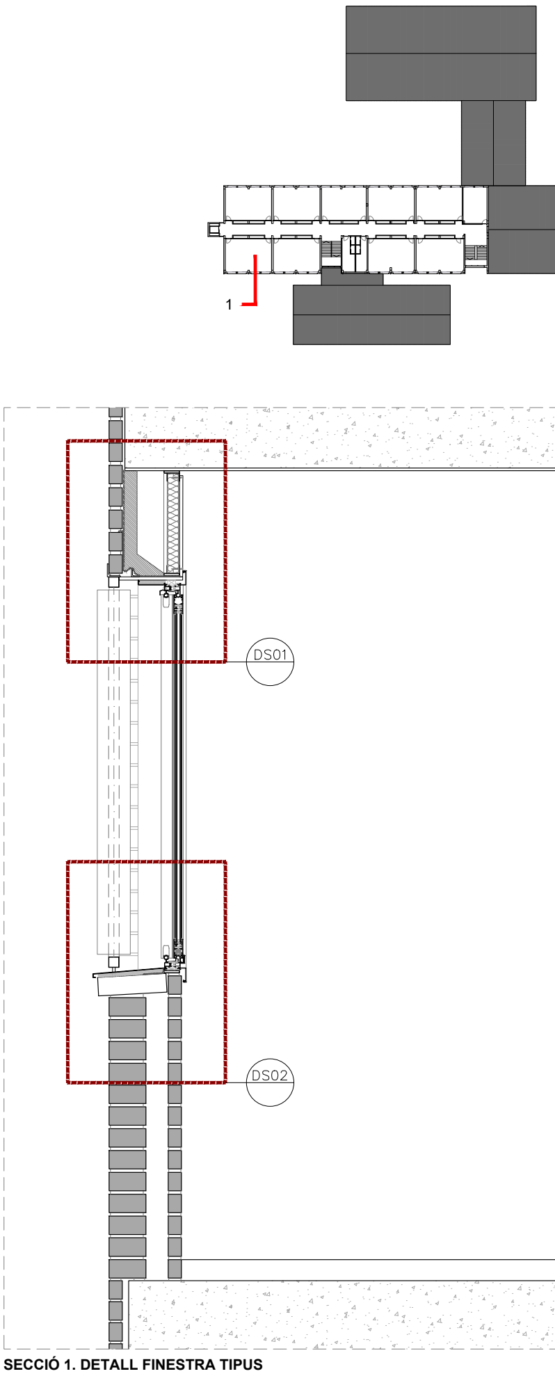
SECCIÓ 1. DETALL FINESTRA TIPUS
