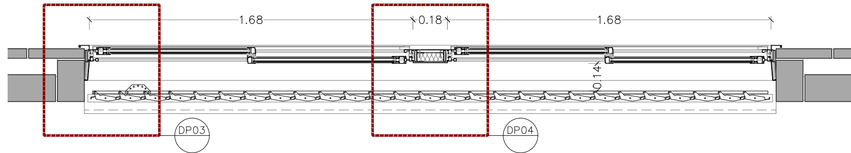
PLANTA FINESTRA TIPUS
