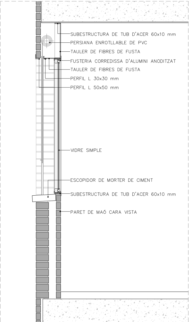
SECCIÓ 1. DETALL FINESTRA TIPUS
