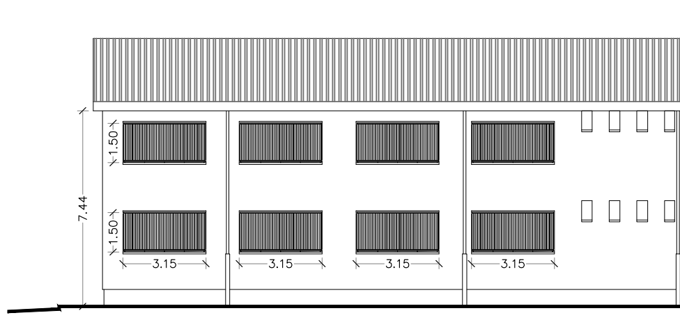
ALÇAT NORD B. GELOSIES
