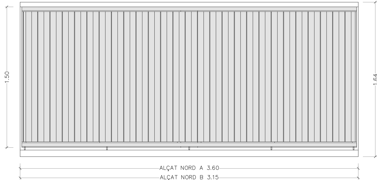
ALÇAT FINESTRA TIPUS. GELOSIA
