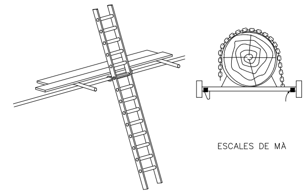
SUBJECCIÓ EN LA PART SUPERIOR
