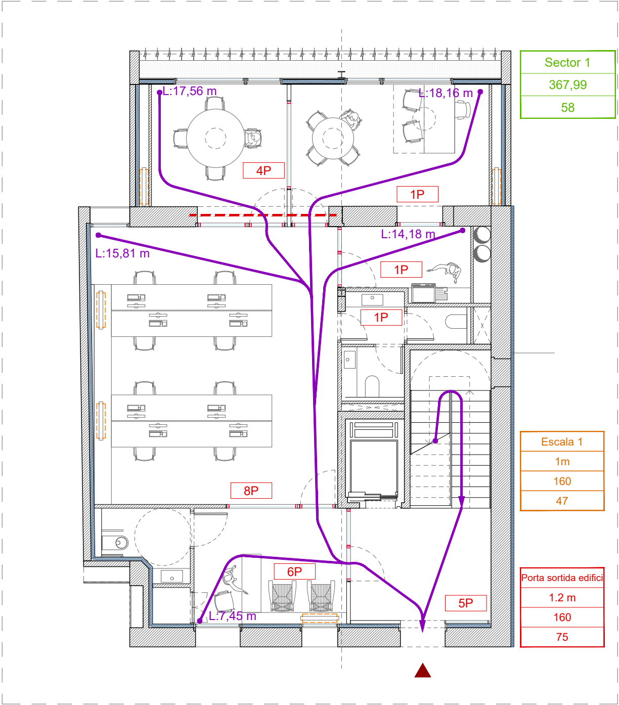
PLANTA BAIXA
