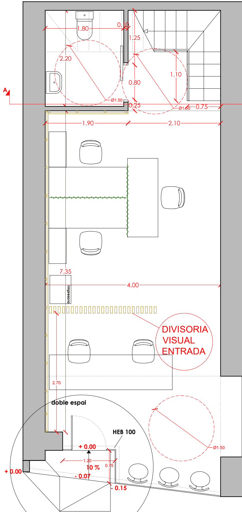
PLANTA BAIXA
