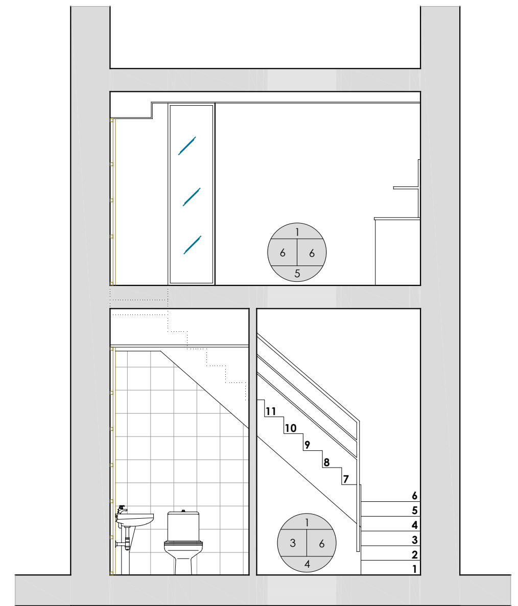
SECCIÓ TRANSVERSAL
