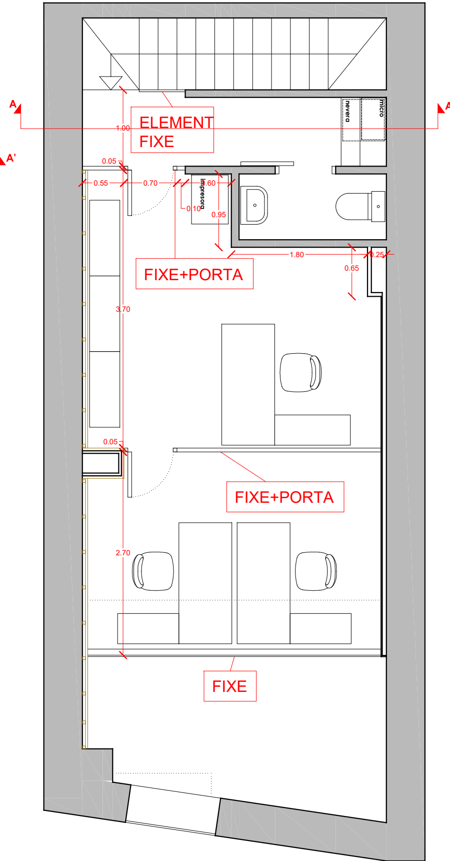
PLANTA ALTELL
