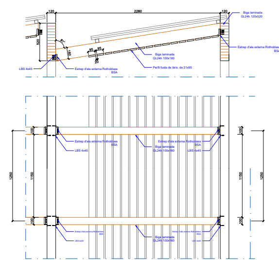
D.3 Detall secció coberta
