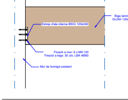
D.5 Detall entrega Jàssera-mur
