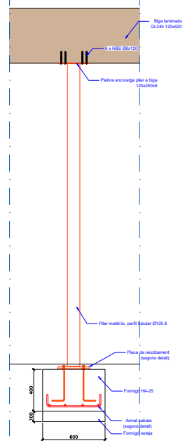
D.4 Detall sabata amb pilar metàl·lic
