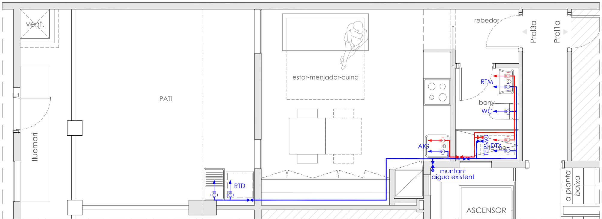
INSTAL·LACIONS - habitatge Pral.3a fontaneria
