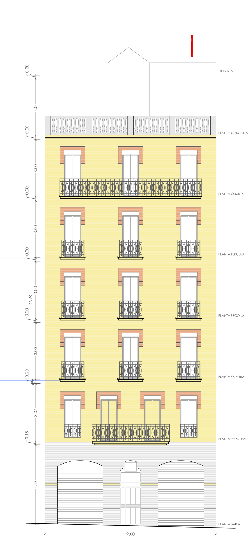
ESTAT ACTUAL - façana principal l·listat d'actuacions
