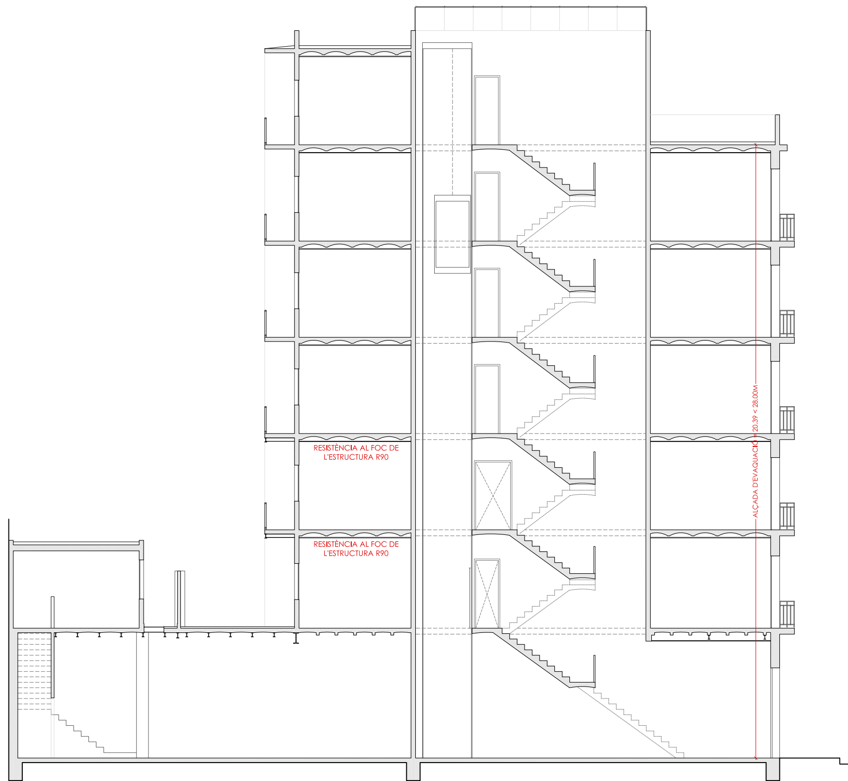
CTE SI - secció longitudinal general seguretat en cas d'incendi
