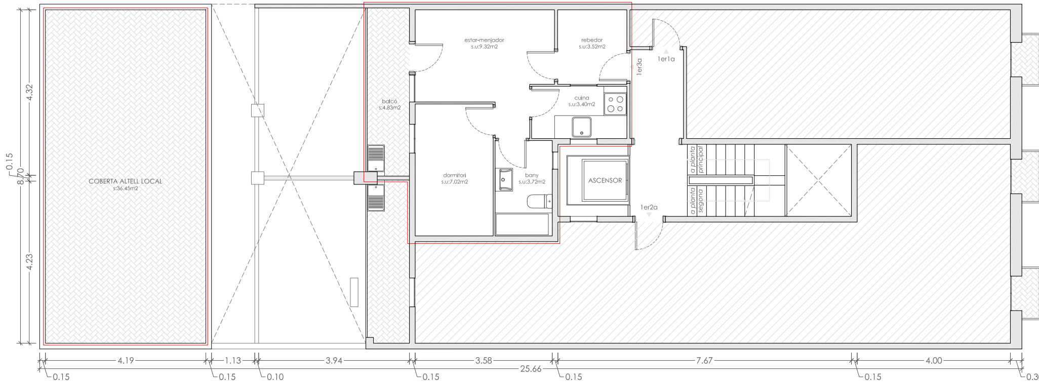
ESTAT ACTUAL - planta primera — àmbit d'intervenció
