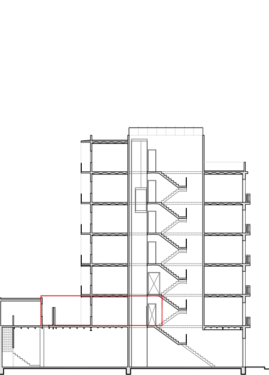
SECCIÓ GENERAL àmbit d'intervenció
