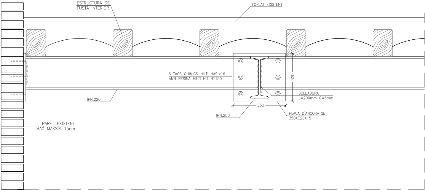
ESTRUCTURA - habitatge Pral.3a detall - reforços tallallums per a control de fletxes
