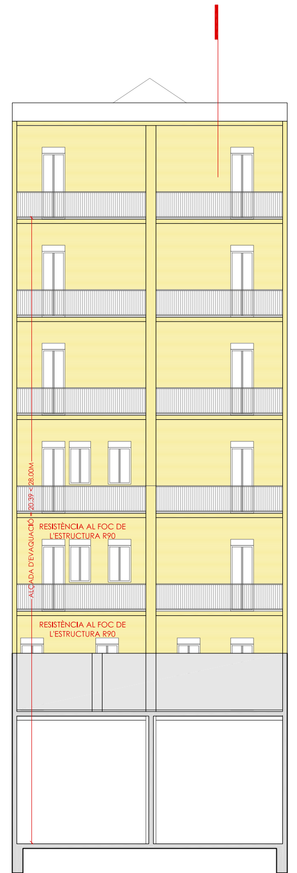
CTE SI - alçat façana posterior seguretat en cas d'incendi
