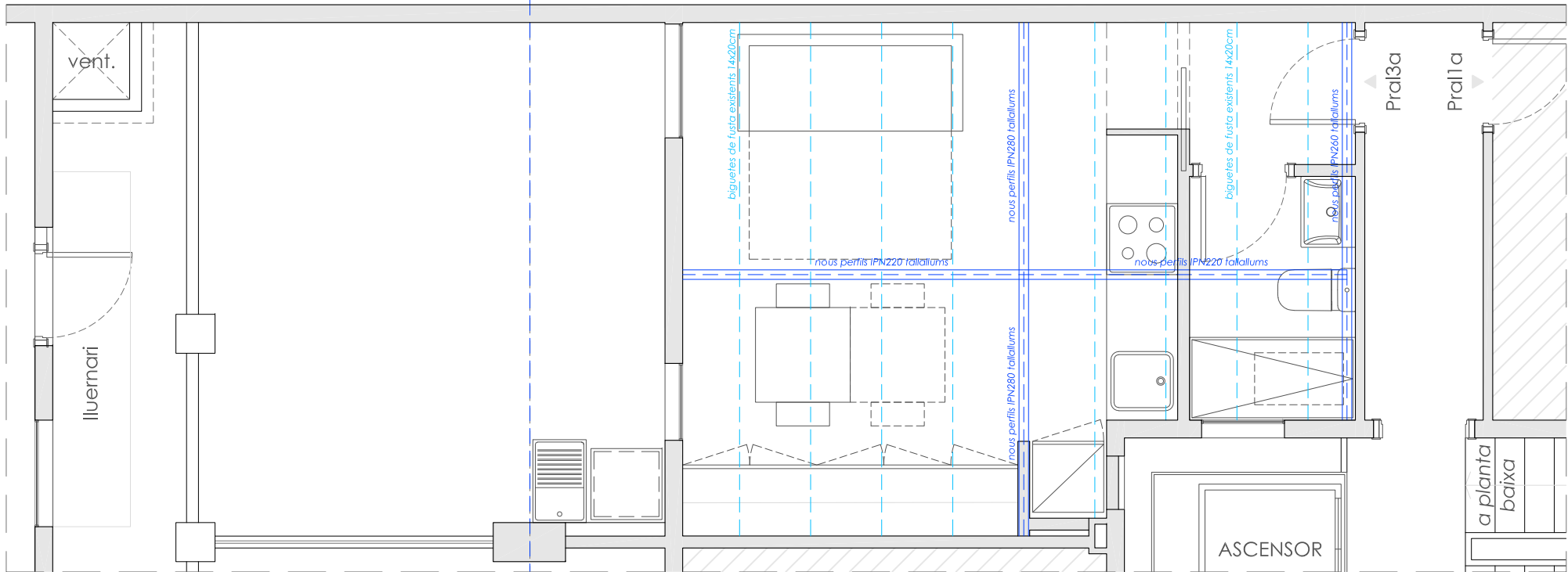
ESTRUCTURA - habitatge Pral.3a planta - reforços tallallums per a control de fletxes
