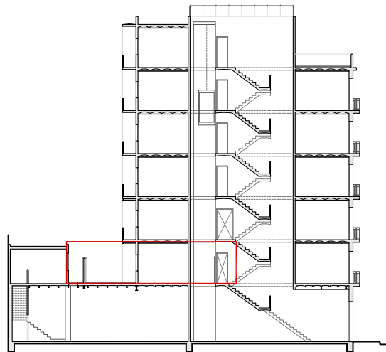
SECCIÓ GENERAL — àmbit d'intervenció
