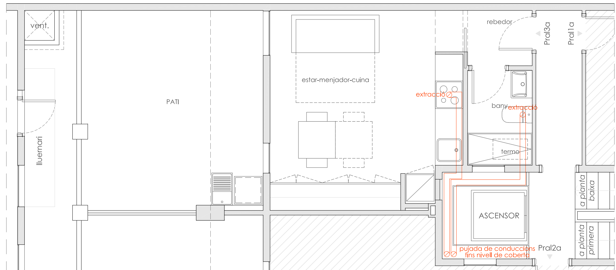
INSTAL·LACIONS - habitatge Pral.3a extracció de fums
