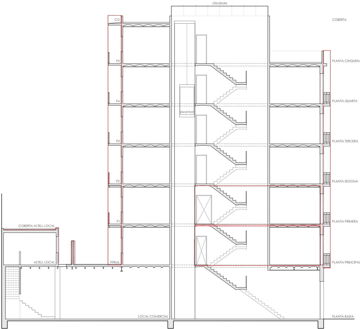
ESTAT ACTUAL - secció longitudinal — àmbit d'intervenció
