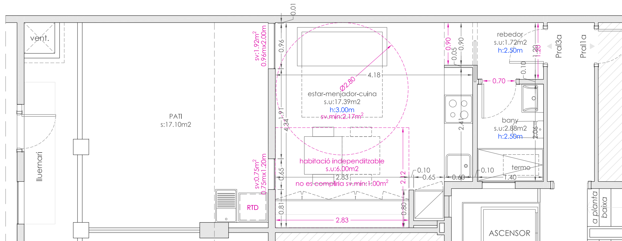
ARQUITECTURA - habitatge Pral.3a superfícies, cotes i D.141/2012
