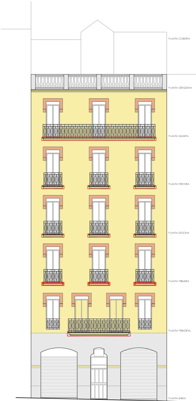
ESTAT ACTUAL - façana principal — àmbit d'intervenció
