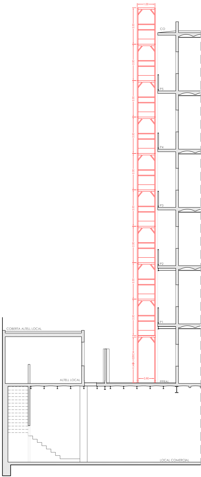
MITJANS AUXILIARS - secció bastida
