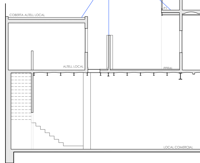
ESTAT ACTUAL - secció l·listat d'actuacions
