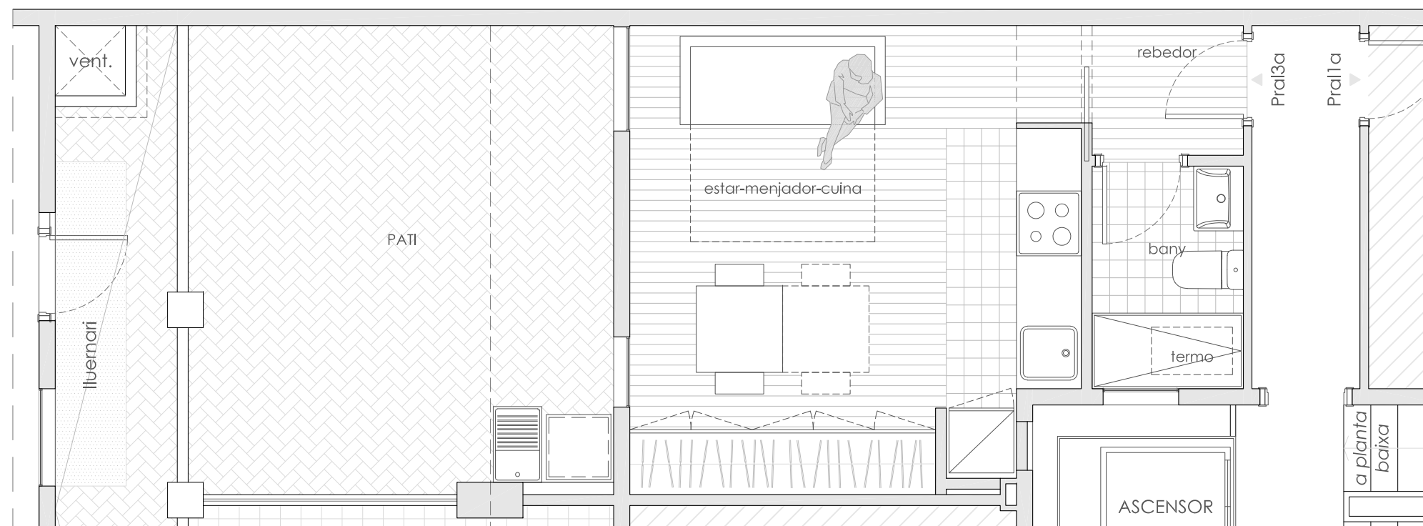
ARQUITECTURA - habitatge Pral.3a distribució
