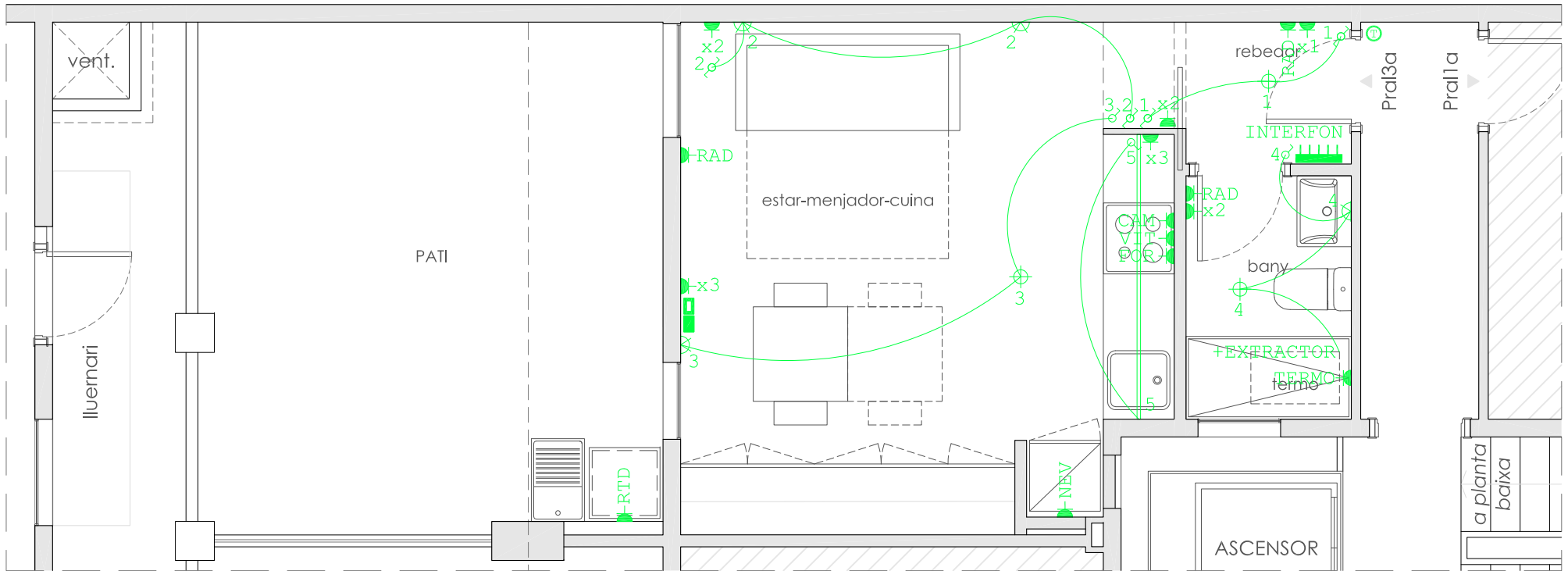
INSTAL·LACIONS - habitatge Pral.3a electricitat
