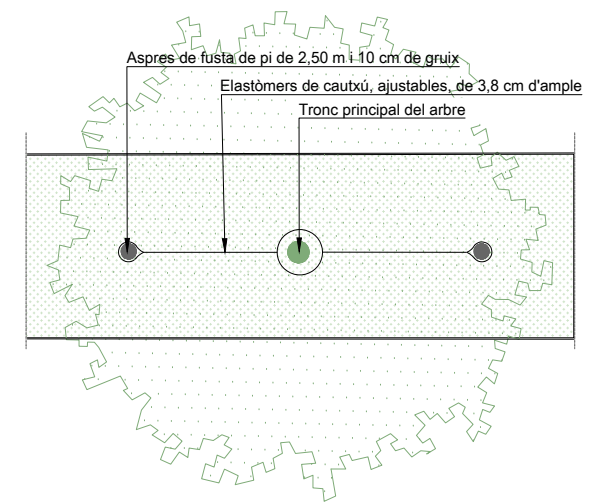
DETALL SUPORT I PROTECCIÓ D'ARBRE Escala 1:50
