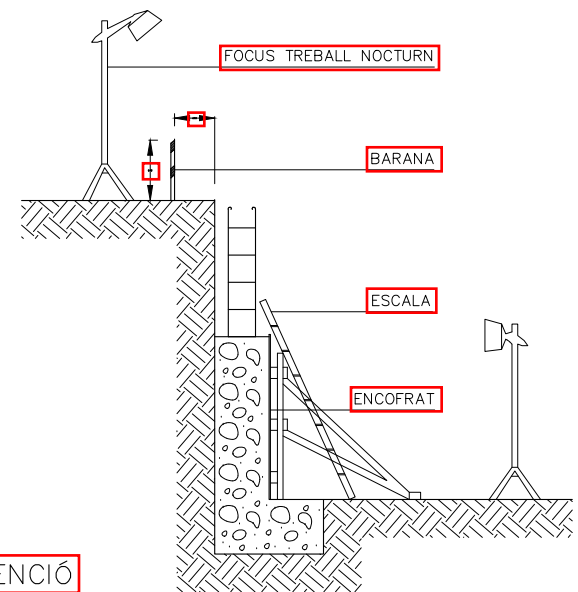
DETALL PÒRTIC BALISAMENT
