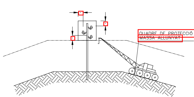
PAS PER SOTA DE LÍNIES AÈRIES DE BAIXA TENSIÓ
