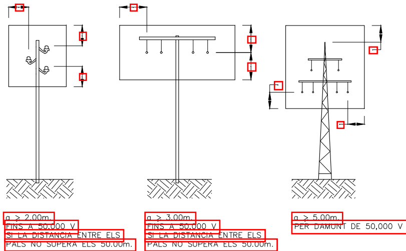
RÈGLES RELATIVES A LA POSTA EN OBRA DE MÀQUINES PROPERES A LÍNIES ELÈCTRIQUES AÈRIES
