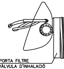
MATERIAL ELASTÒMER
