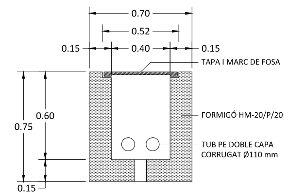
ARQUETA TELECOMUNICACIONS 0,40 x 0,40m interior
