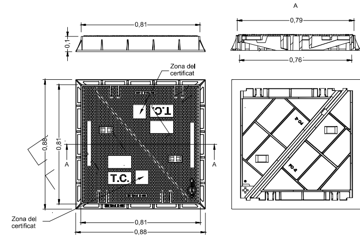
Tapa de fosa D400 Arqueta de telecomunicacions 0,70x0,70m interior
