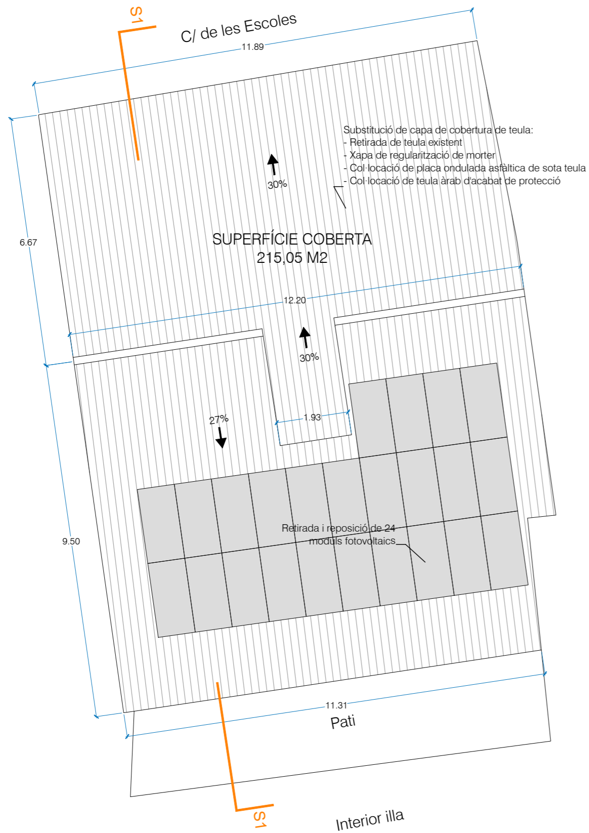
PLANTA COBERTA E:1/100
