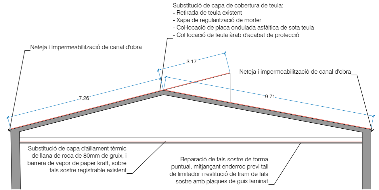
SECCIÓ COBERTA - S1 E:1/100
