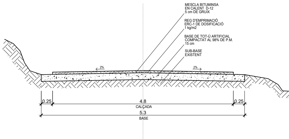
SECCIÓ TIPUS CAMÍ ESCALA 1/50
