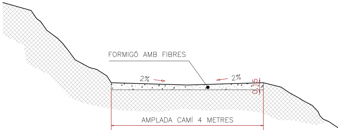
SECCIÓ TRANSVERSAL TIPUS
