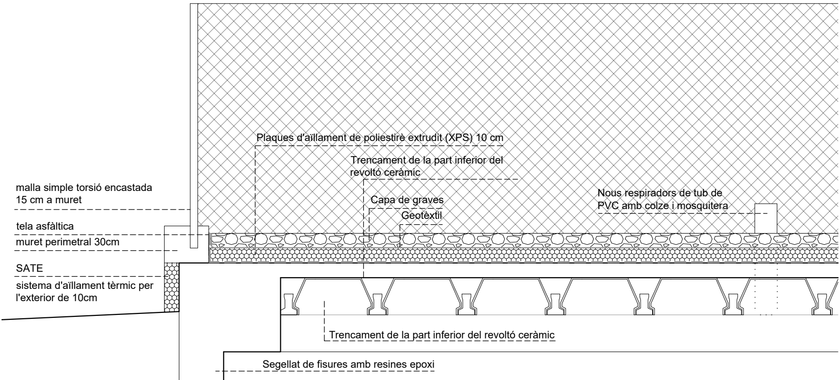
DETALL SECCIÓ A. E 1/25
