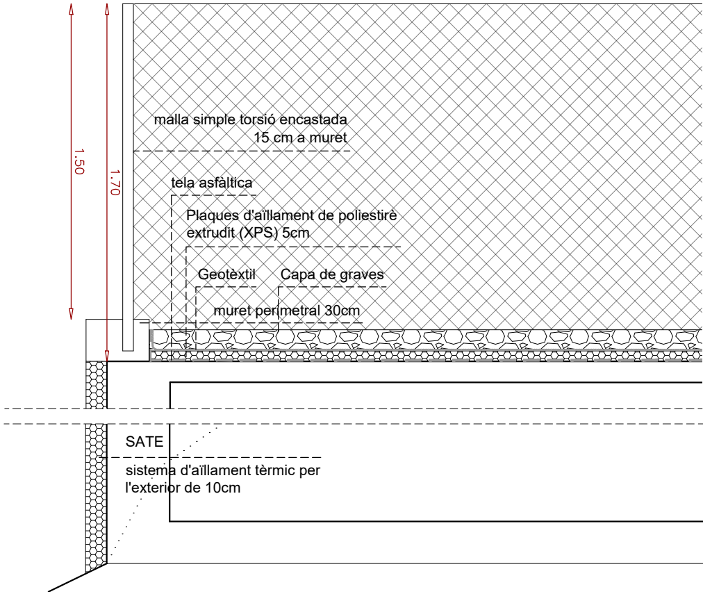
DETALL SECCIÓ B. E 1/25
