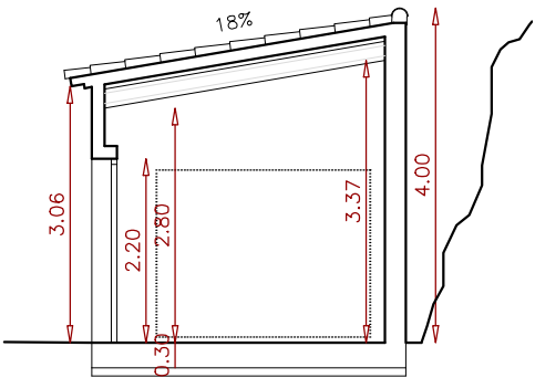
SECCIÓ TRANSVERSAL A
