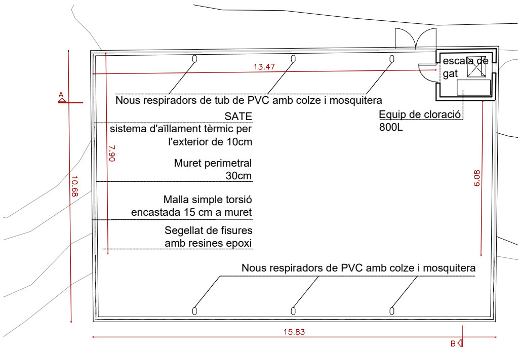
PLANTA COBERTA
