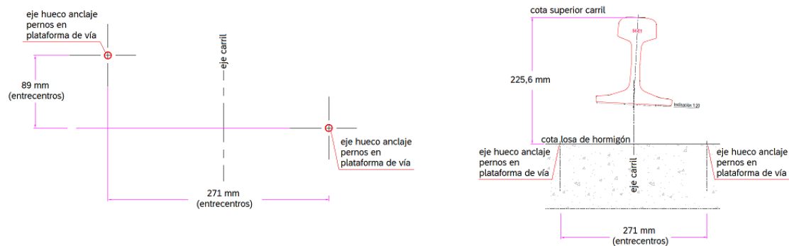
Imatge 1. Detall evolutiu fixació sense suport de contracarril. Font: elaboració pròpia.
