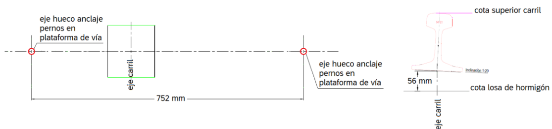
Imatge 2. Detall evolutiu fixació amb suport de contracarril. Font: elaboració pròpia.
