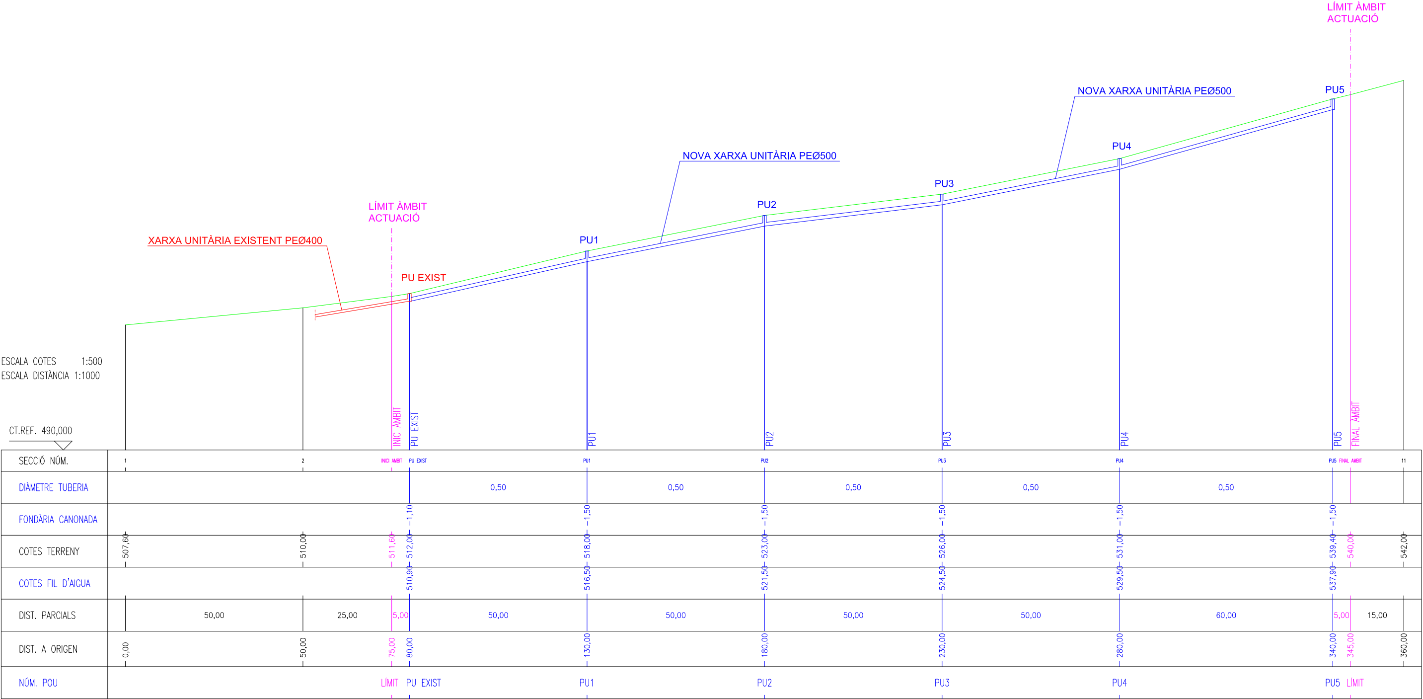
PERFIL CLAVEGUERAM UNITARI CARRER DEL NORD NÚM. 3 I EL CARRER DEL MIGDIA NÚMERO 4 DE CAN PRAT
