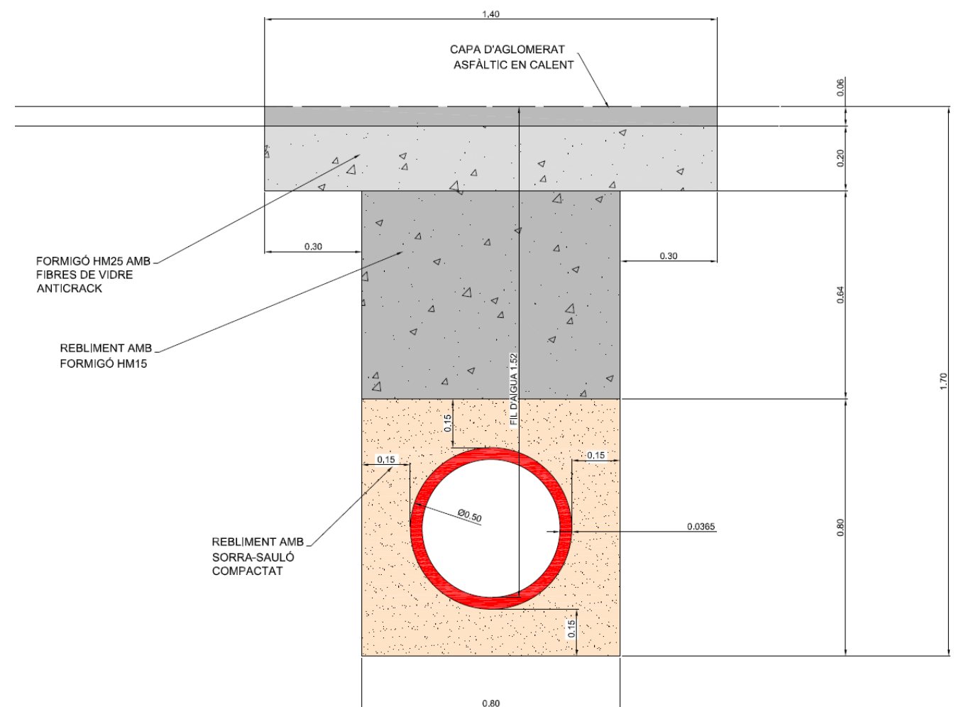
Imatge 1. Secció tipus rasa clavegueram
