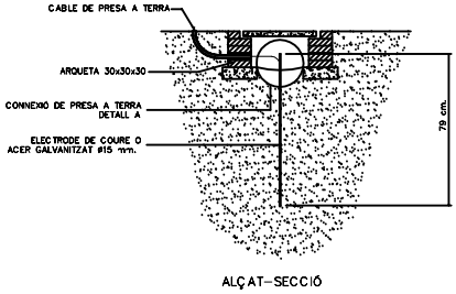
PRESA A TERRA NORMALITZADA GENERAL DE L' OBRA RESISTÈNCIA 80 OHMS, RESISTIVITAT 50 M. OHMS
