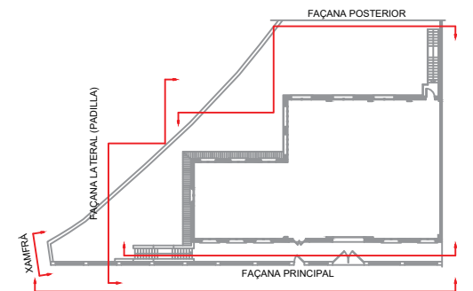
PLANTA BAIXA
