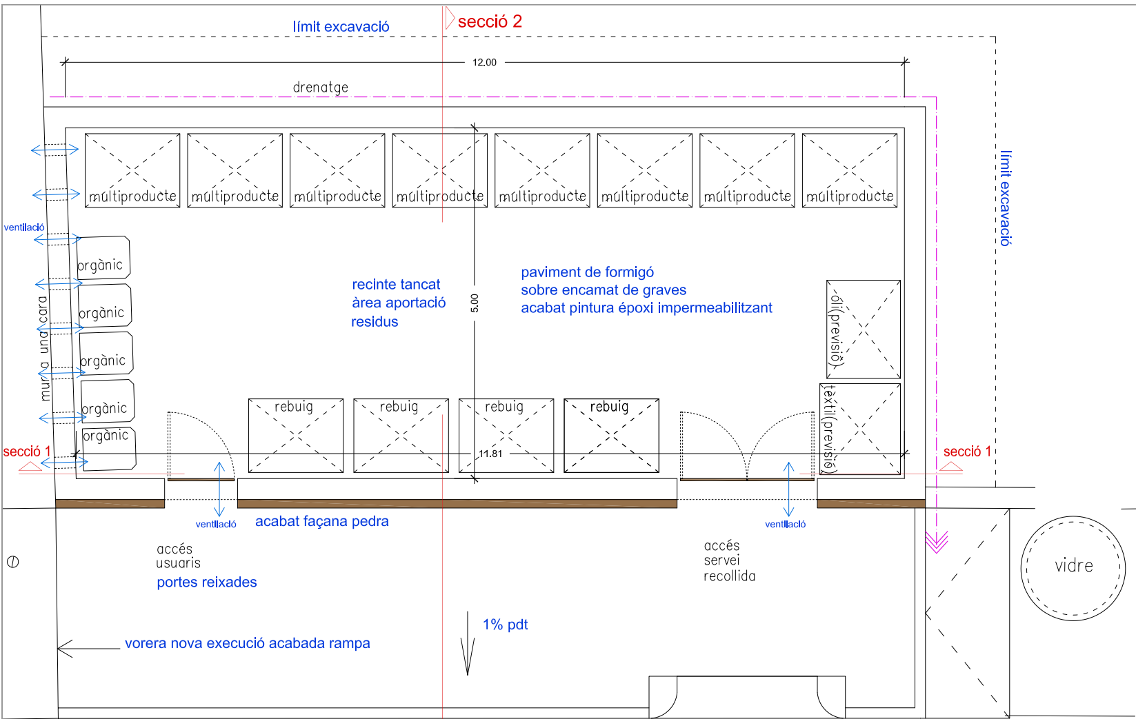
PLANTA DE DISTRIBUCIÓ
