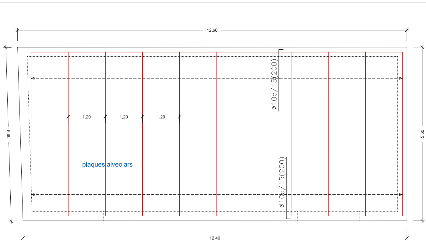
PLANTA FORJAT SOSTRE
