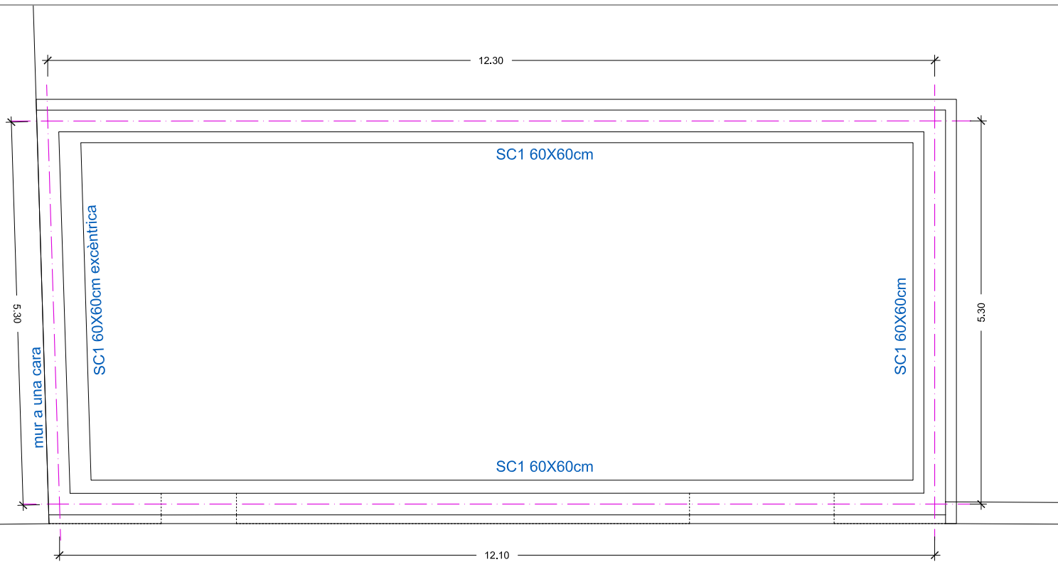
PLANTA DE FONAMENTACIÓ
