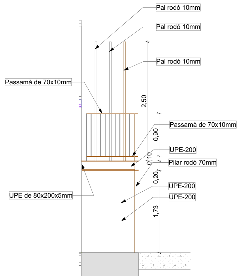
VISTA C-C
