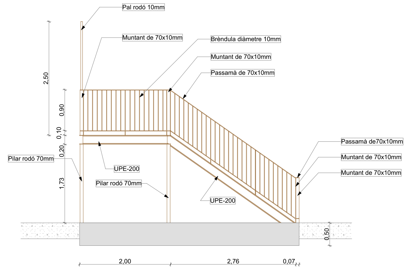
VISTA A-A
