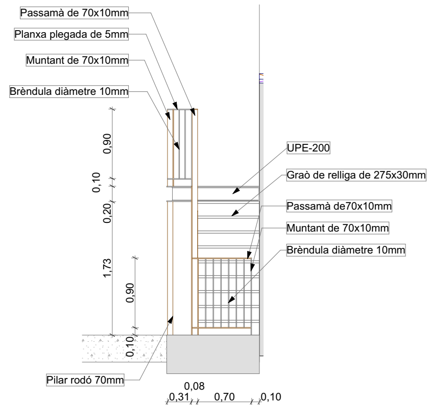
VISTA D-D
