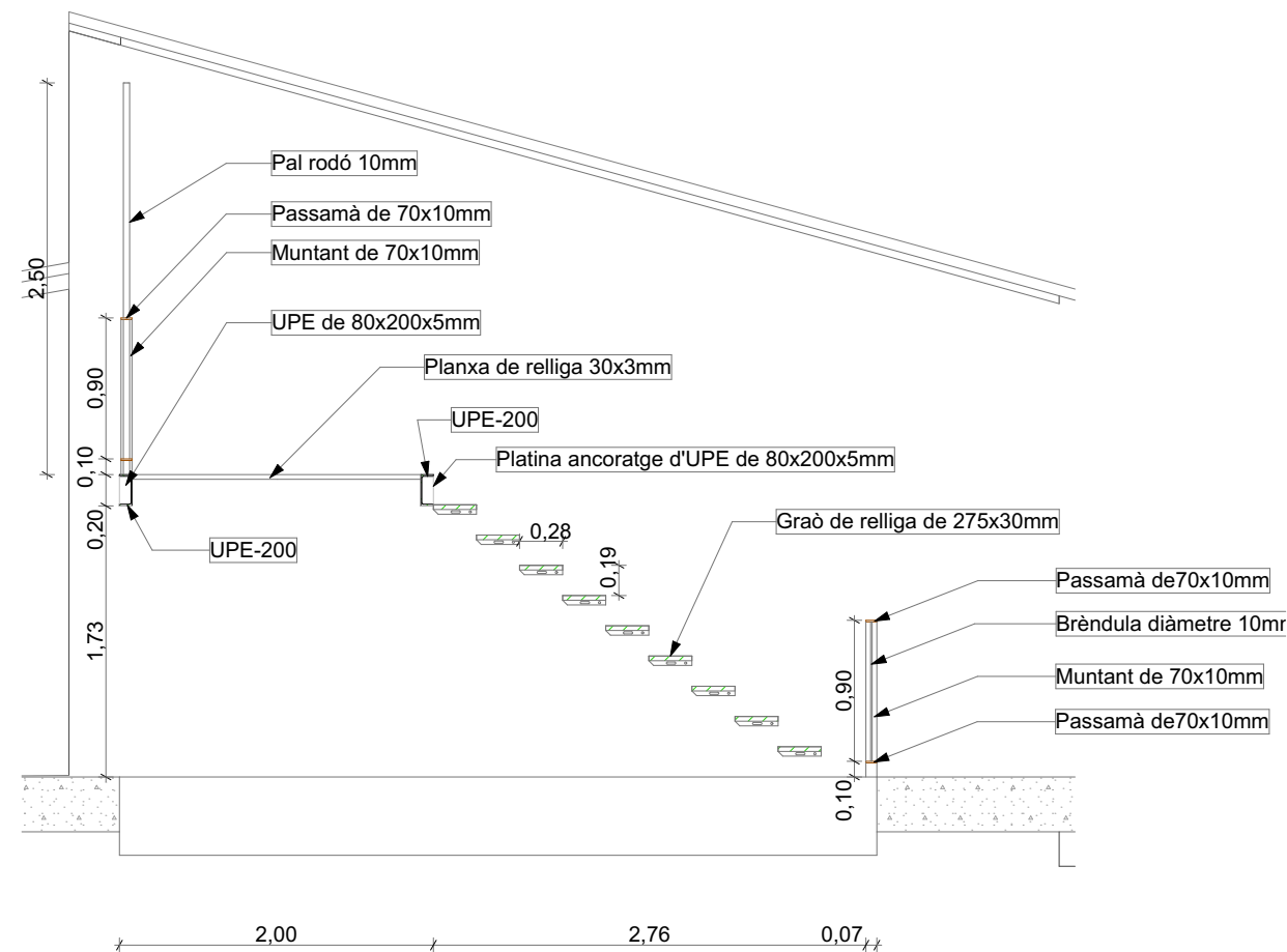
VISTA B-B
