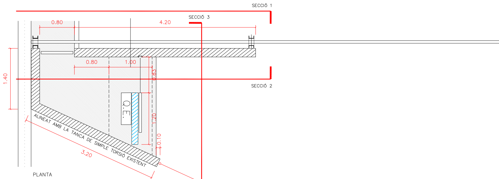
PLANTA
