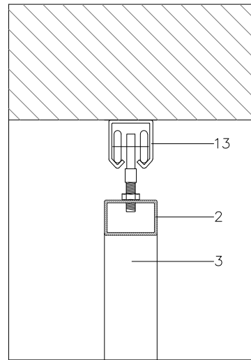
DETALL 4
