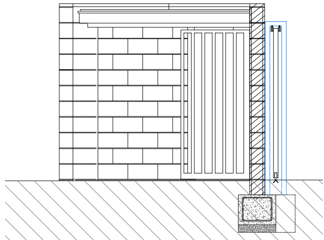
SECCIÓ 3
