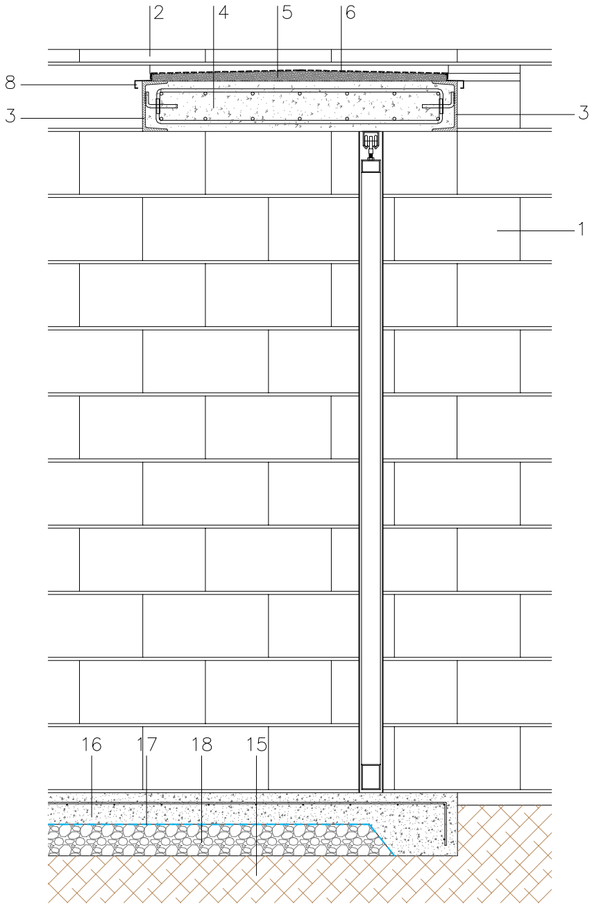
SECCIÓ CONSTRUCTIVA 1
