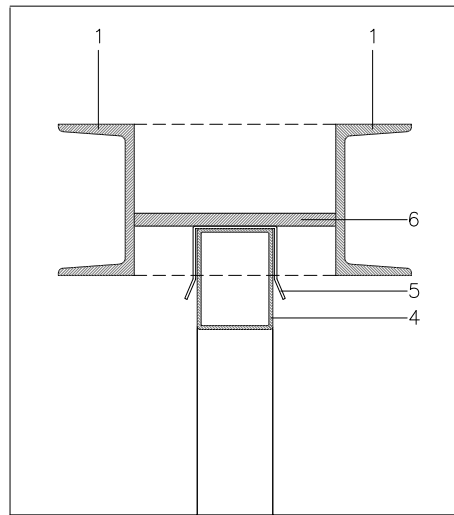
DETALL 3
