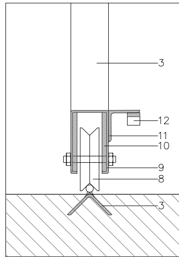
DETALL 2
