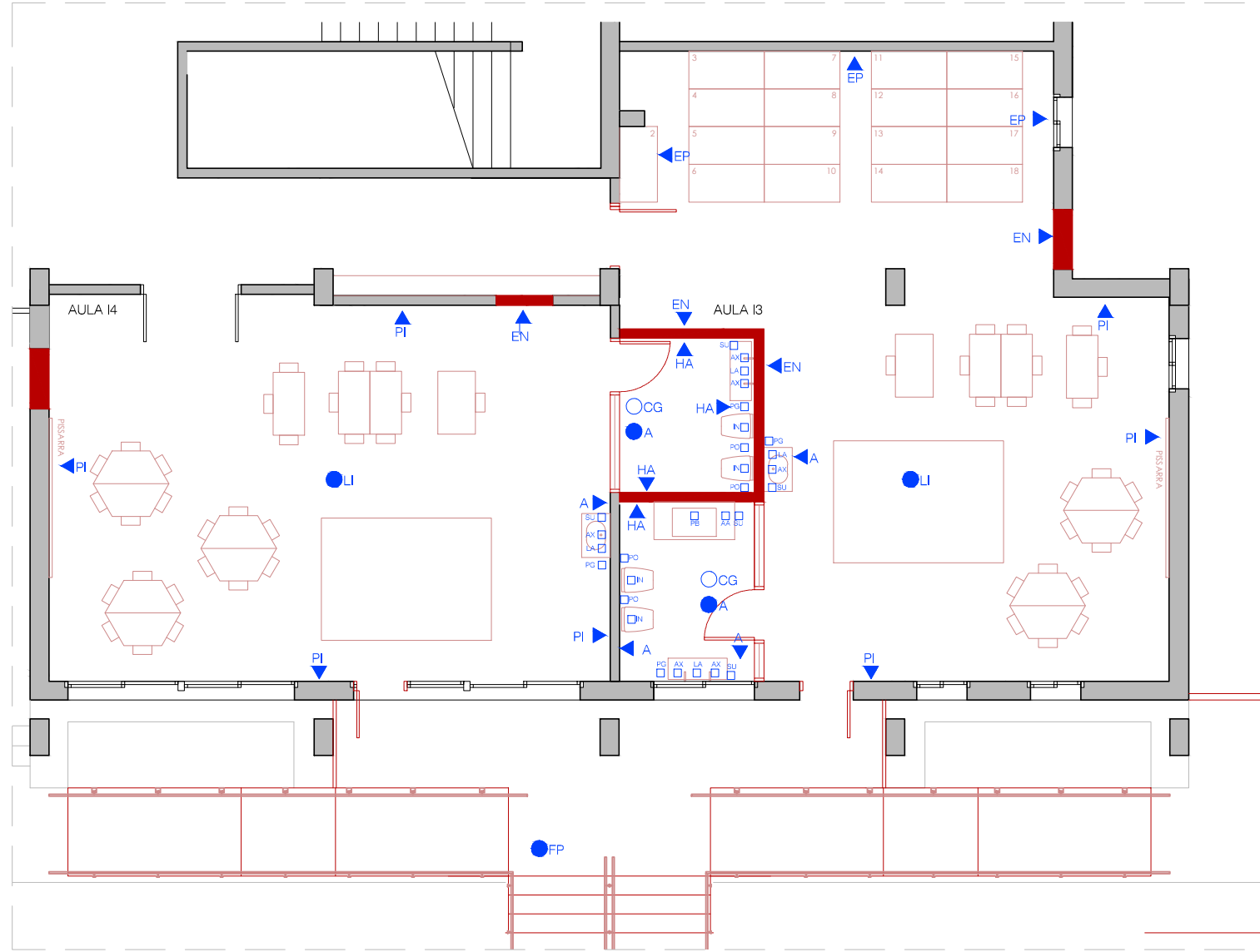
Planta baixa zoom 0.B
