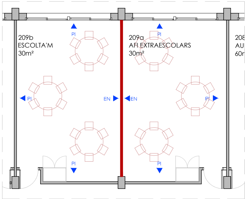
Planta segona zoom 2.A
