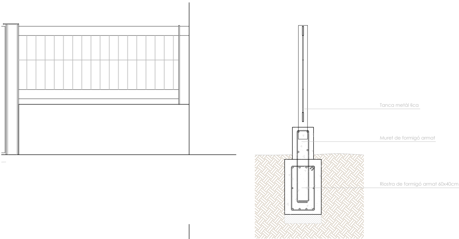
Detall fonamentació murets E: 1/25
