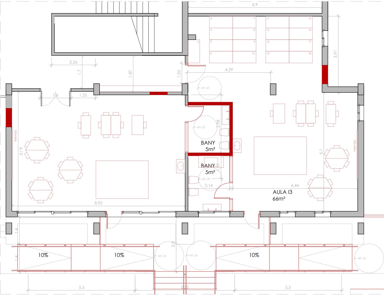
Planta baixa zoom 0.B
