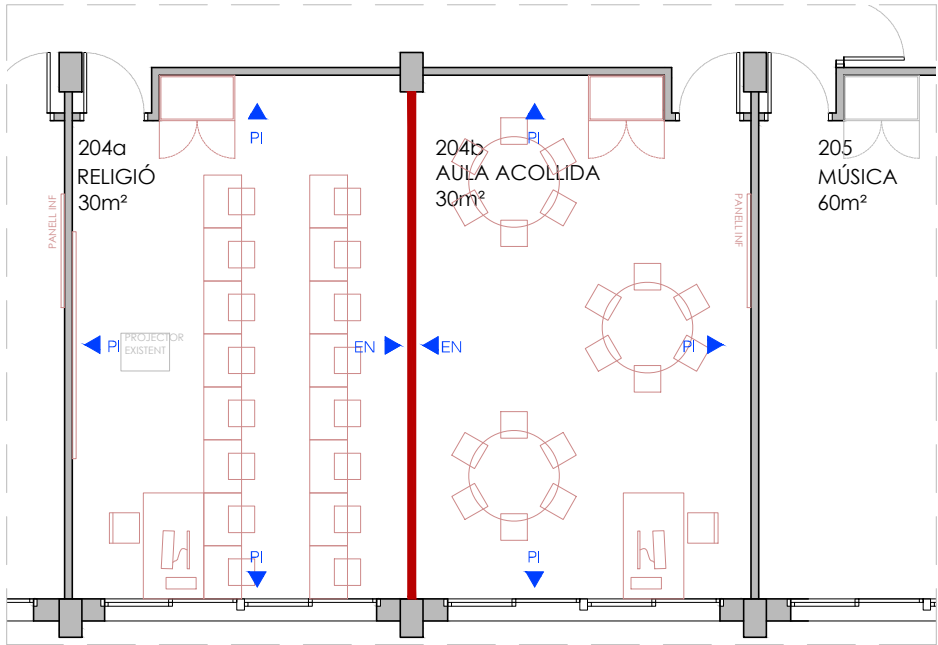
Planta segona zoom 2.B
