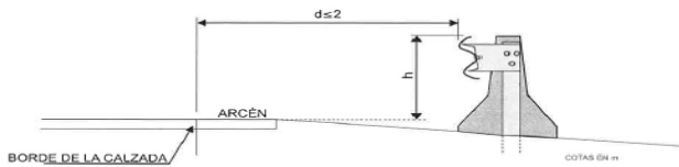
FIGURA 13. DISPOSICIÓN EN ALTURA DE LAS BARRERAS DE SEGURIDAD SITUADAS A MENOS DE 2m DEL BORDE DE LA CALZADA.
