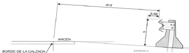
FIGURA 14. DISPOSICIÓN EN ALTURA DE LAS BARRERAS DE SEGURIDAD SITUADAS A MÁS DE 2m DEL BORDE DE LA CALZADA.
