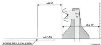
FIGURA 10. DISTANCIA MÍNIMA ENTRE UN SISTEMA DE CONTENCIÓN DE VEHÍCULOS Y UN OBSTÁCULO (d s ).
