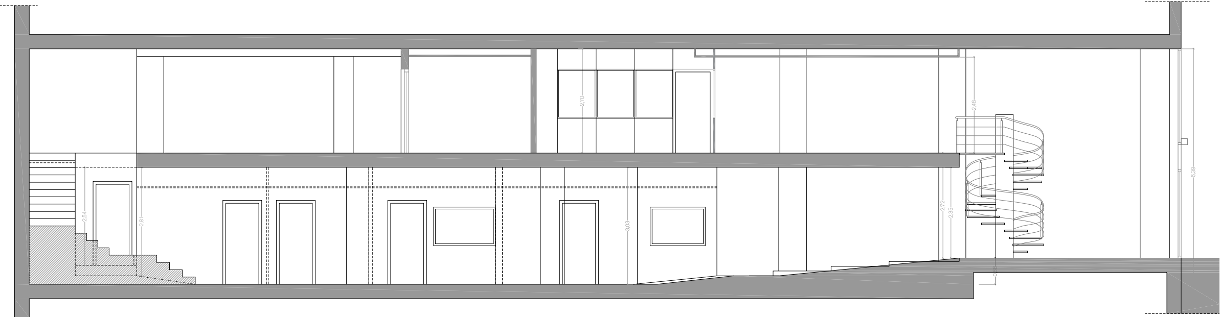
SECCIÓ A
