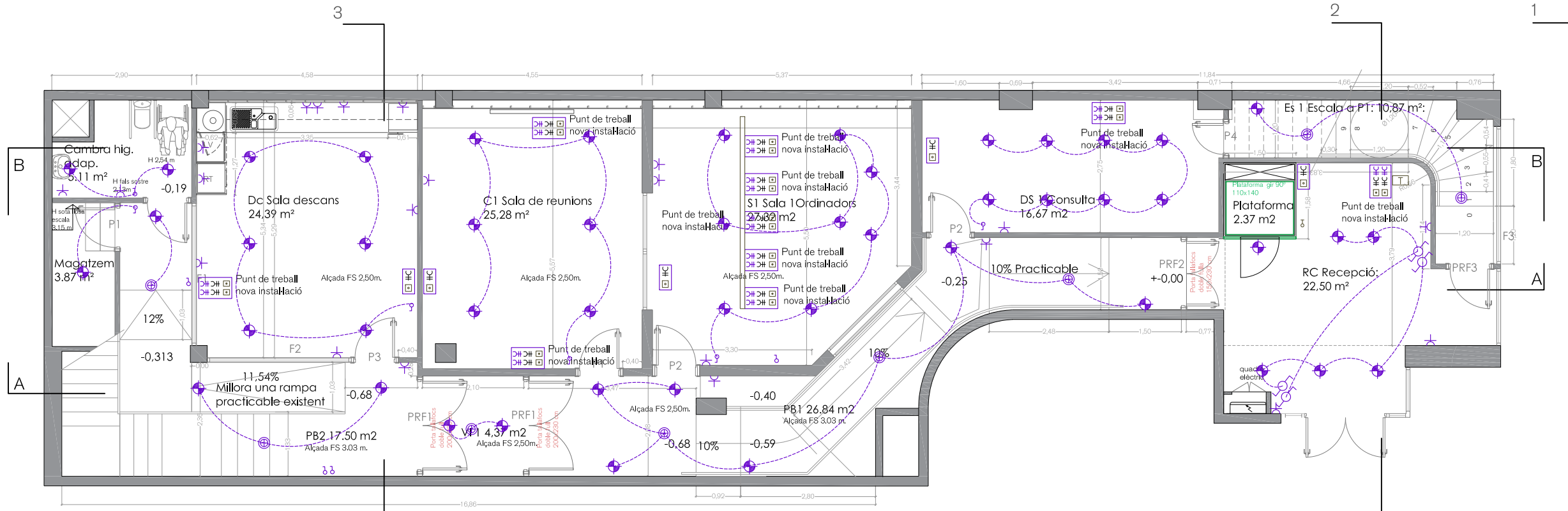
PLANTA BAIXA
