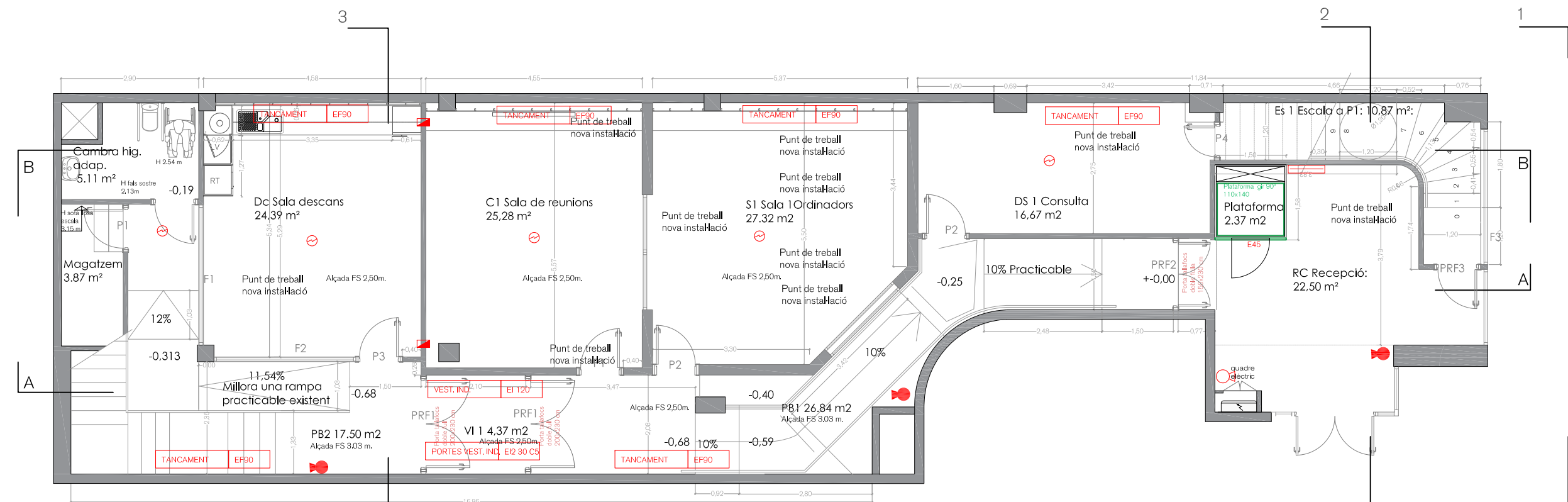
PLANTA BAIXA
