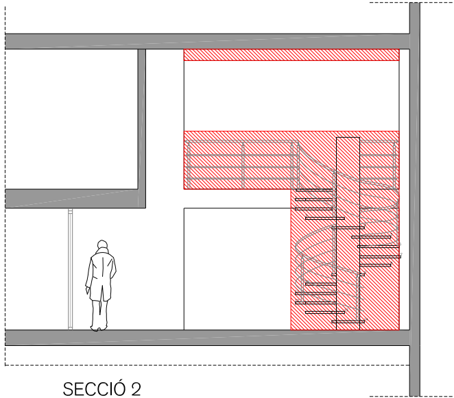
SECCIÓ 2
