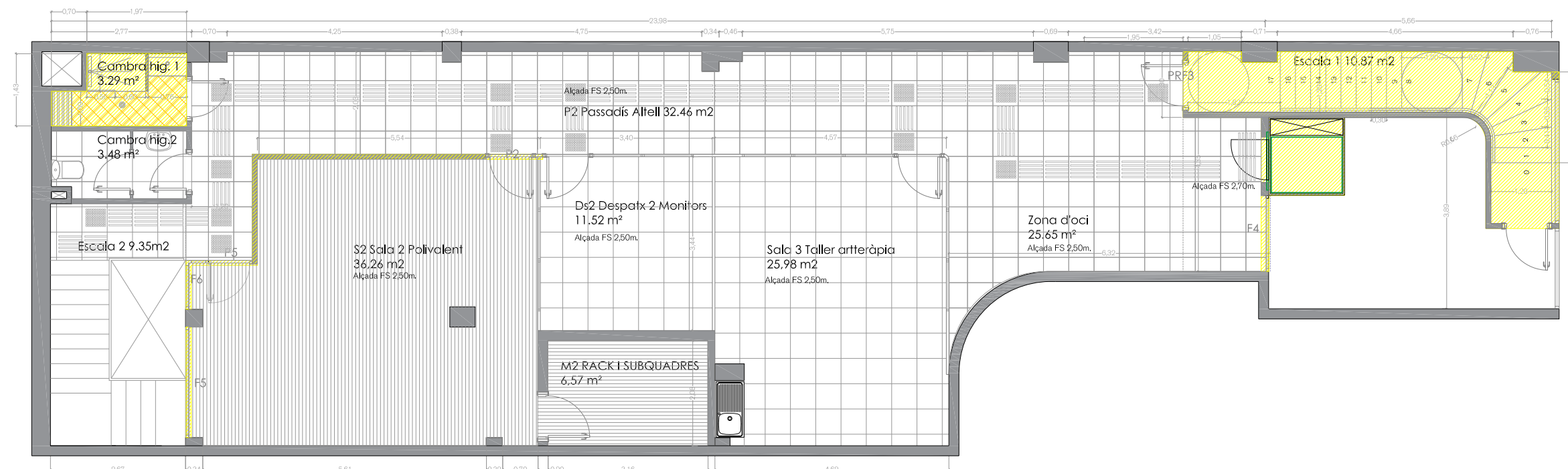
PLANTA ALTELL
