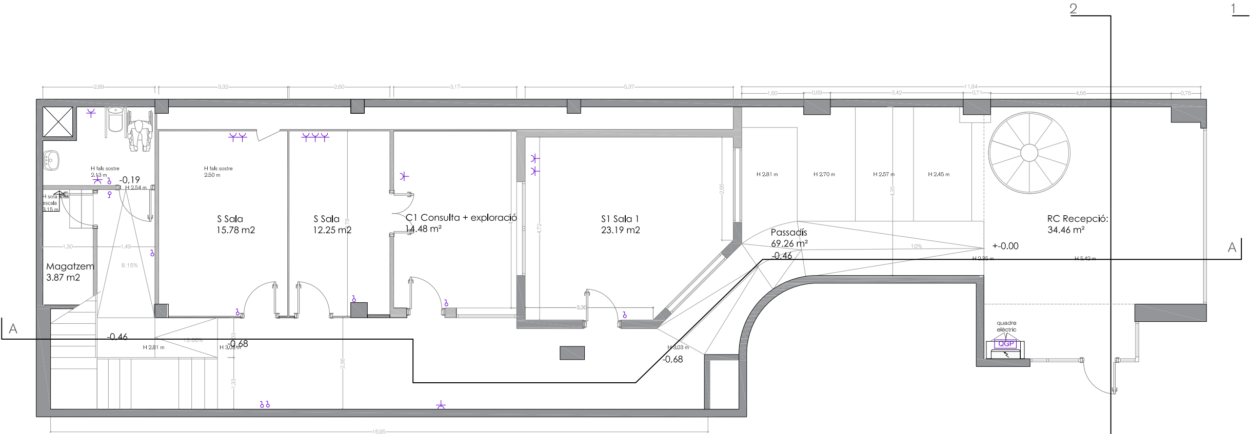
PLANTA BAIXA
