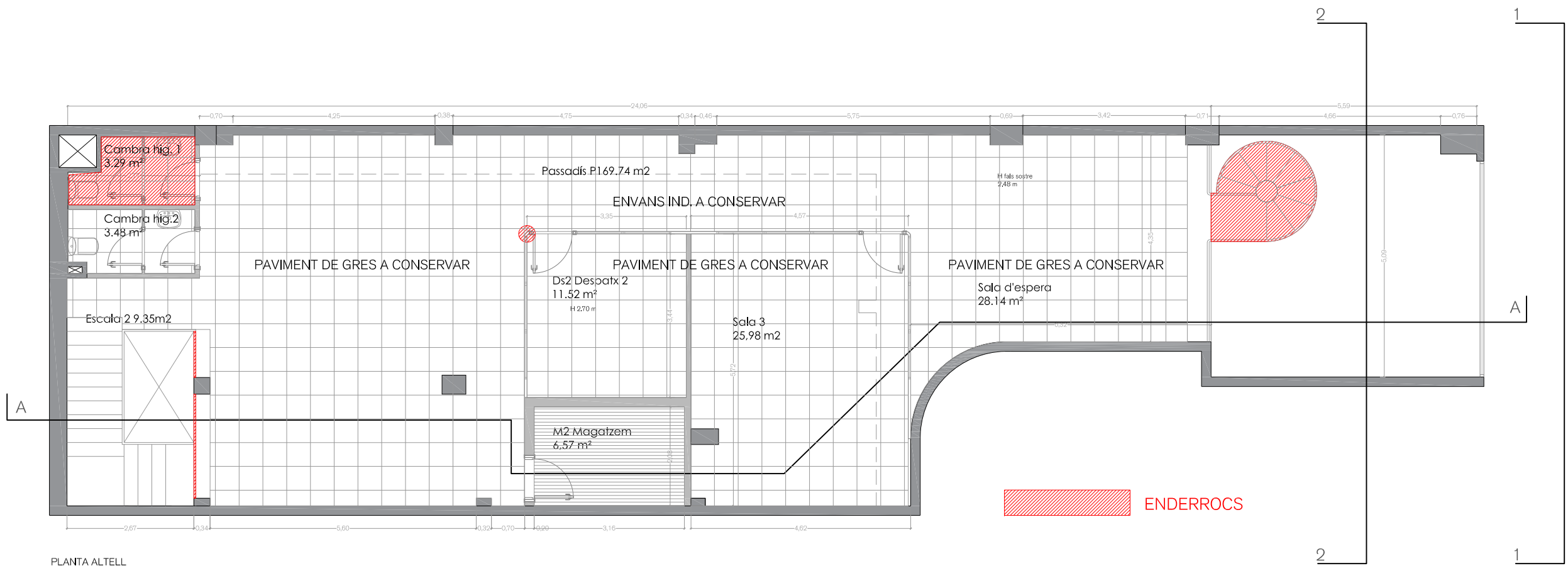
PLANTA ALTELL
