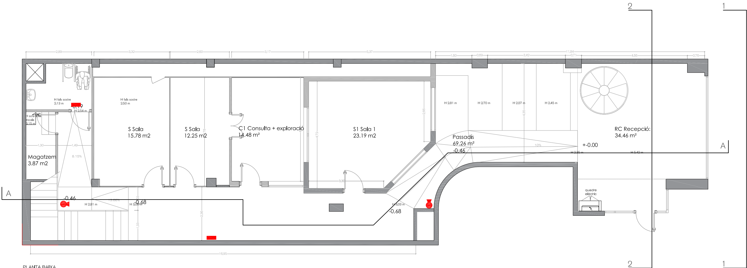
PLANTA BAIXA
