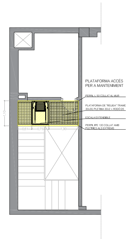
PLANTA ALTELL
