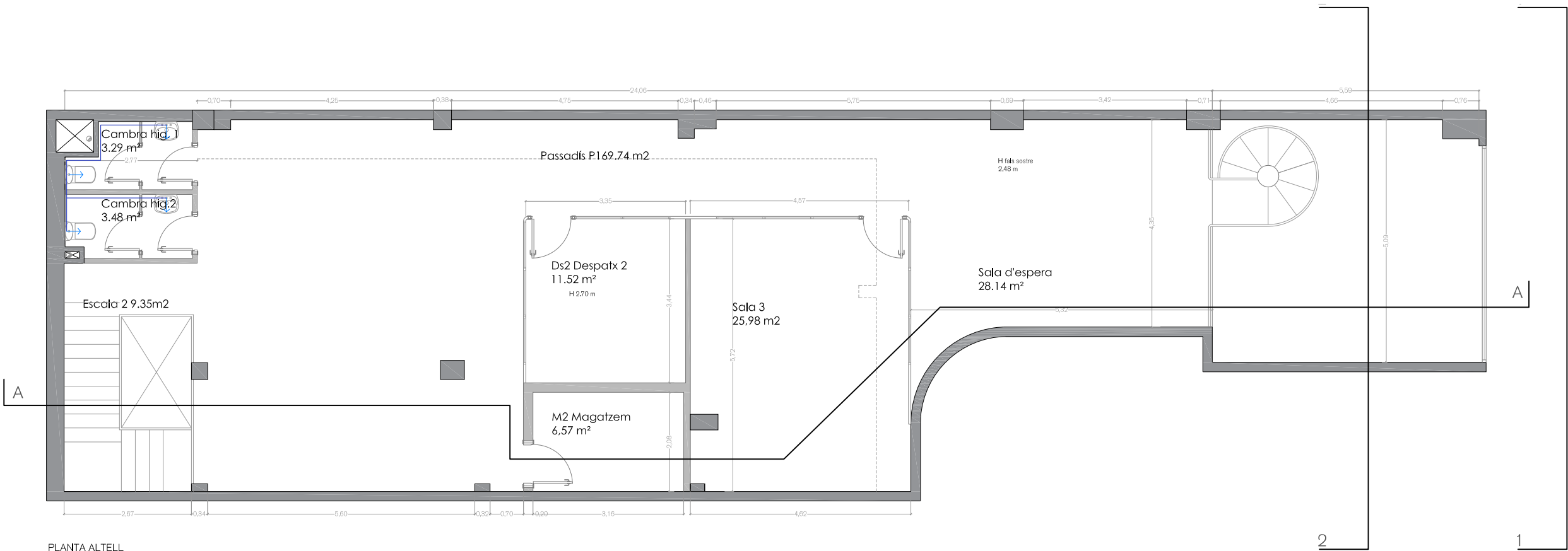
PLANTA ALTELL
