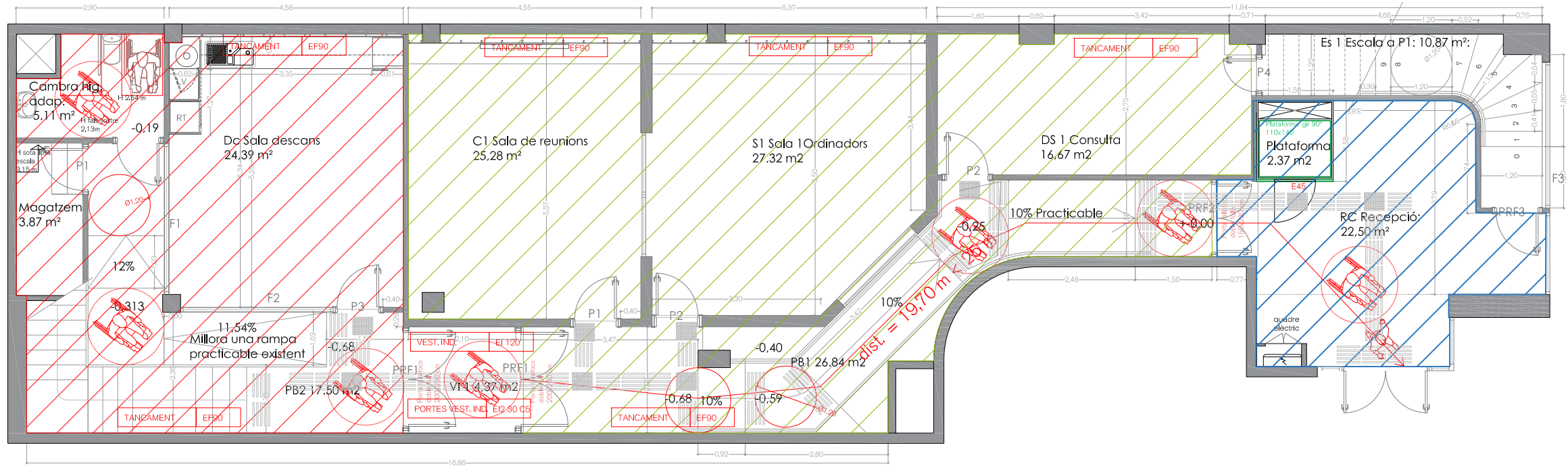
PLANTA BAIXA
