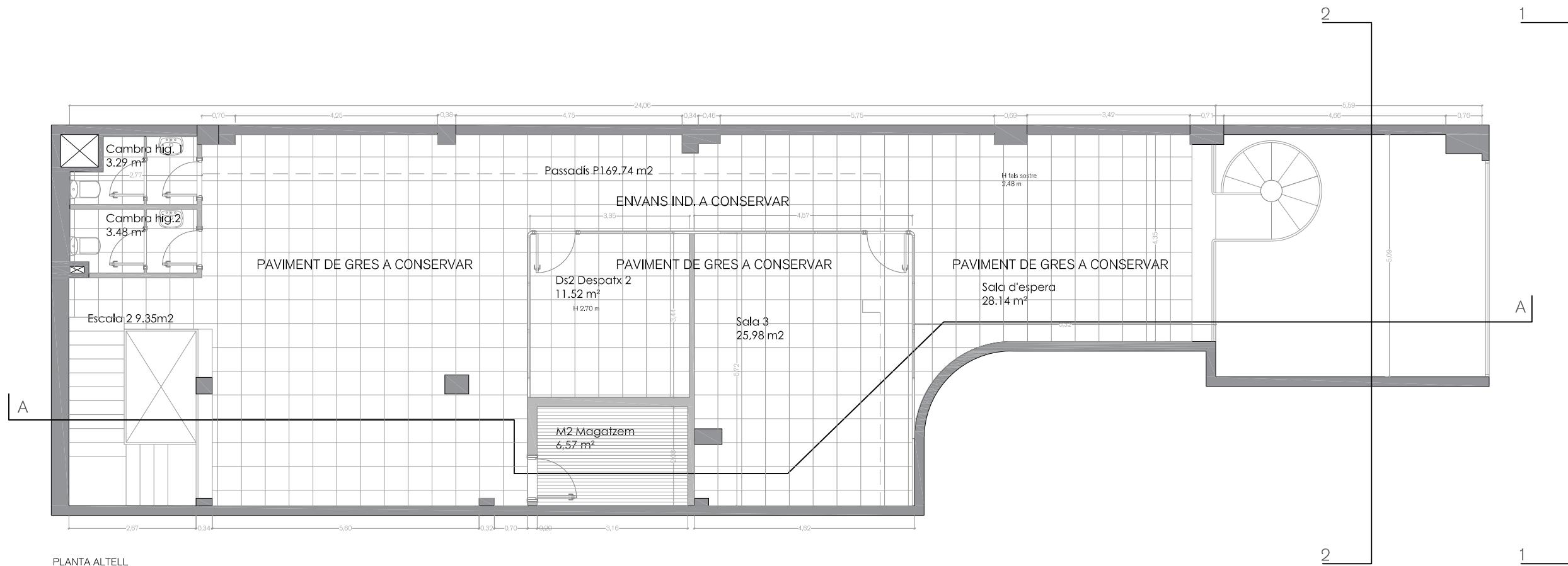
PLANTA ALTELL
