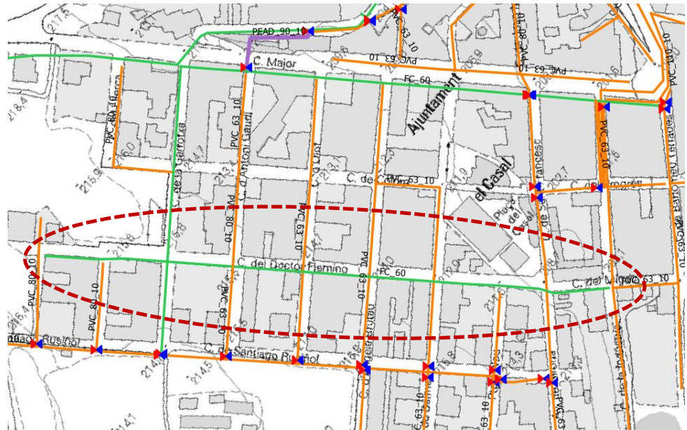
Figura 2.- Plànol extret del pla director. En verd la canonada de fibrociment
