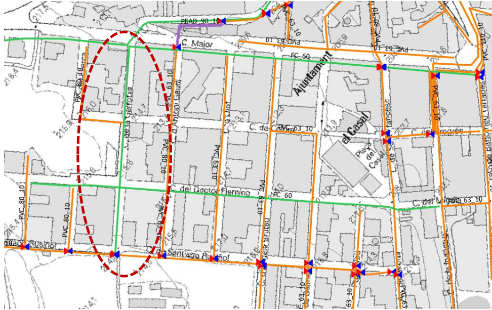
Figura 1.- Plànol extret del pla director. En verd la canonada de fibrociment
