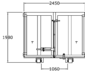
2 HOJAS APERTURA FORMA LIBRO
