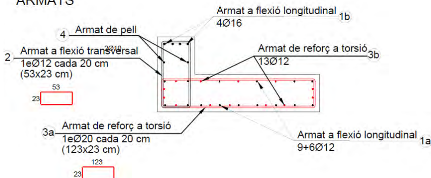
Dimensions i armats d'impоста lateral
