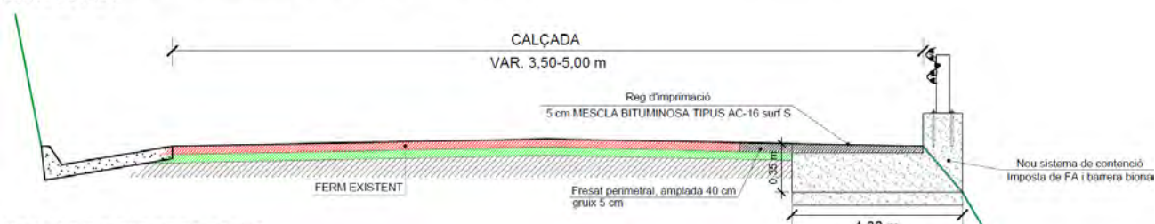
Secció tipus de vial amb imposta lateral.
