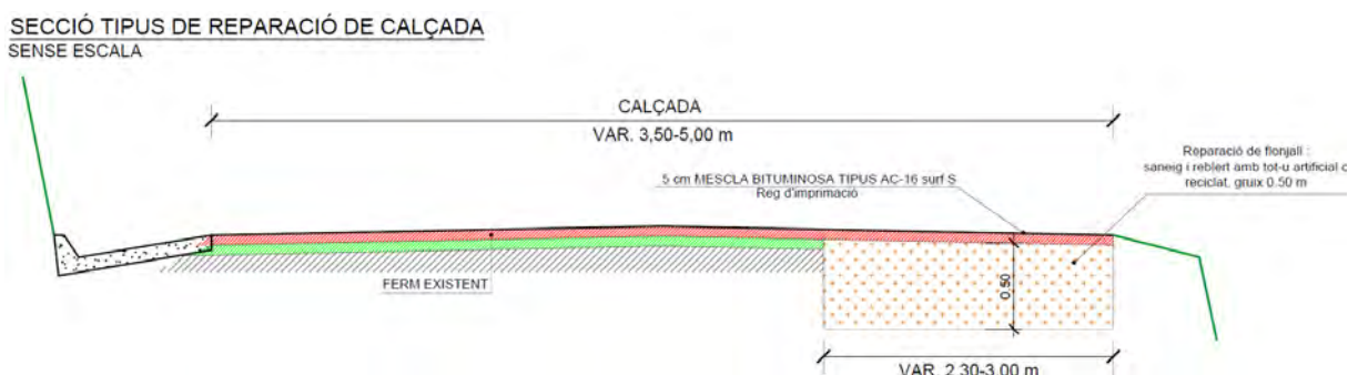
Secció tipus de vial reparat.
