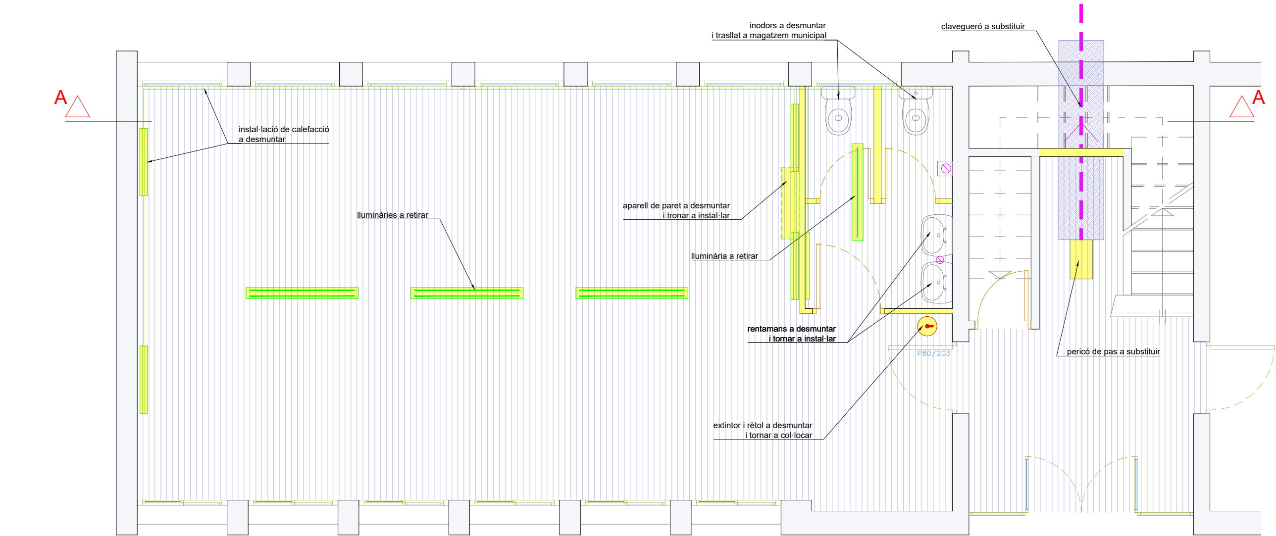
EDIFICI 3 aula i5 - Planta baixa
