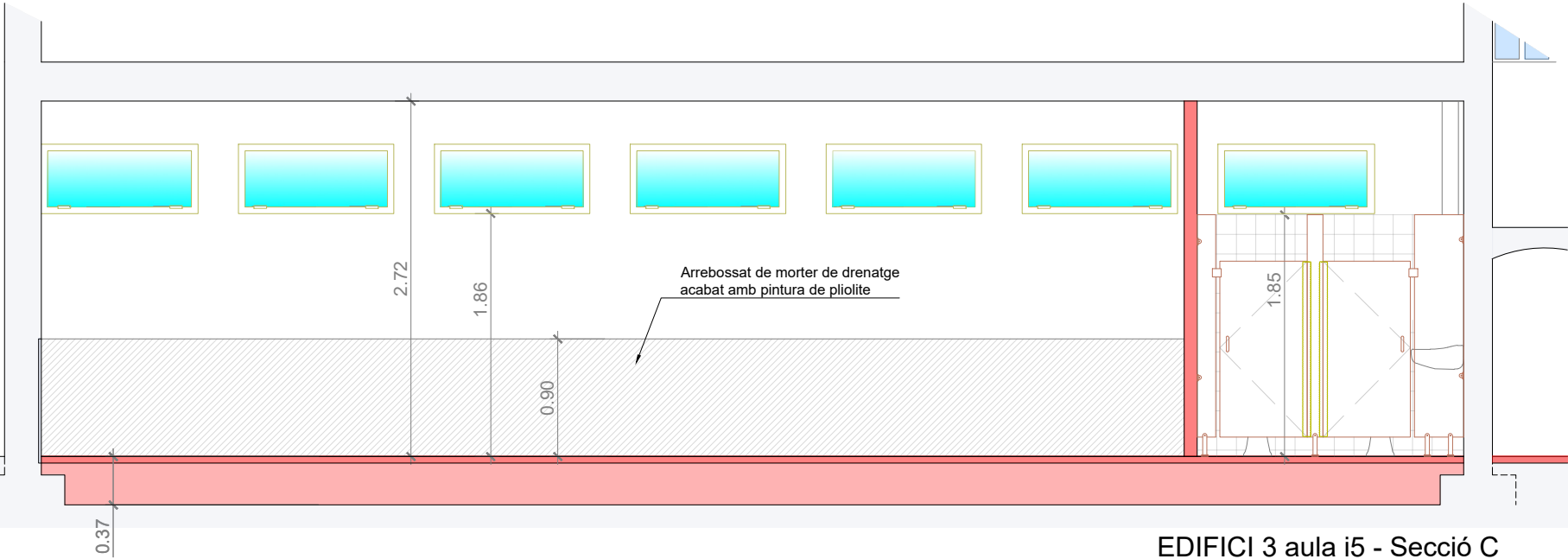
EDIFICI 3 aula i5 - Secció C
