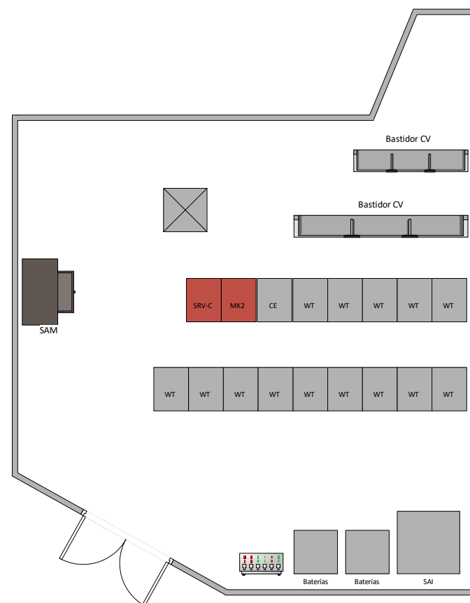
Figura 5. Distribució d'equips proposada per a l'enclavament de Vall d'Hebron.
