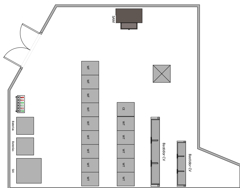
Figura 3. Distribució d'equips actual de l'enclavament de Vall d'Hebron.
