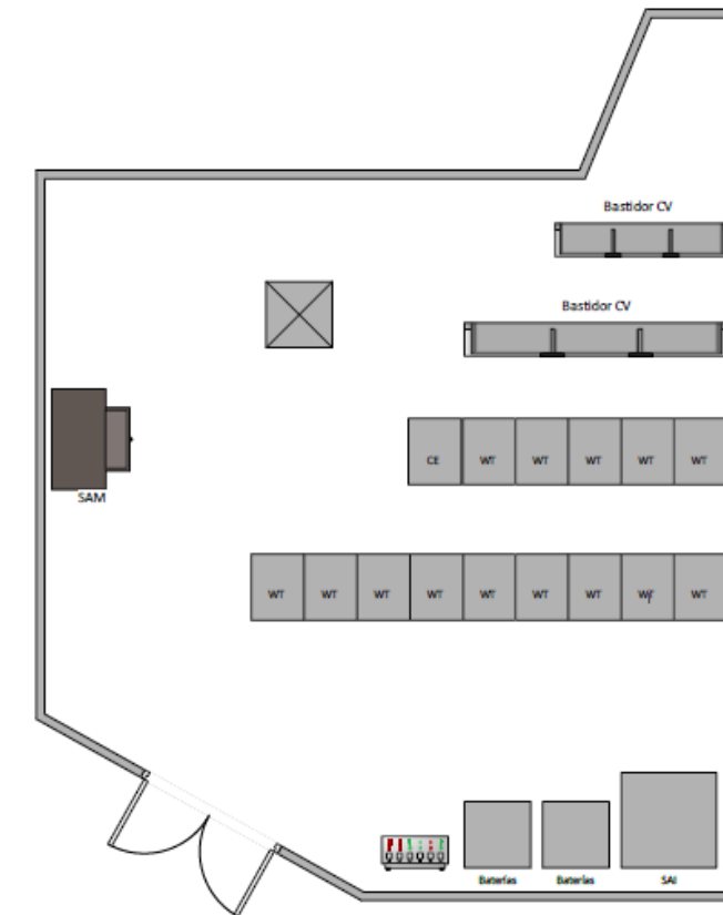
Figura 3 Distribució d'equips actual i'enclavament de Vall d'Hebrón.
