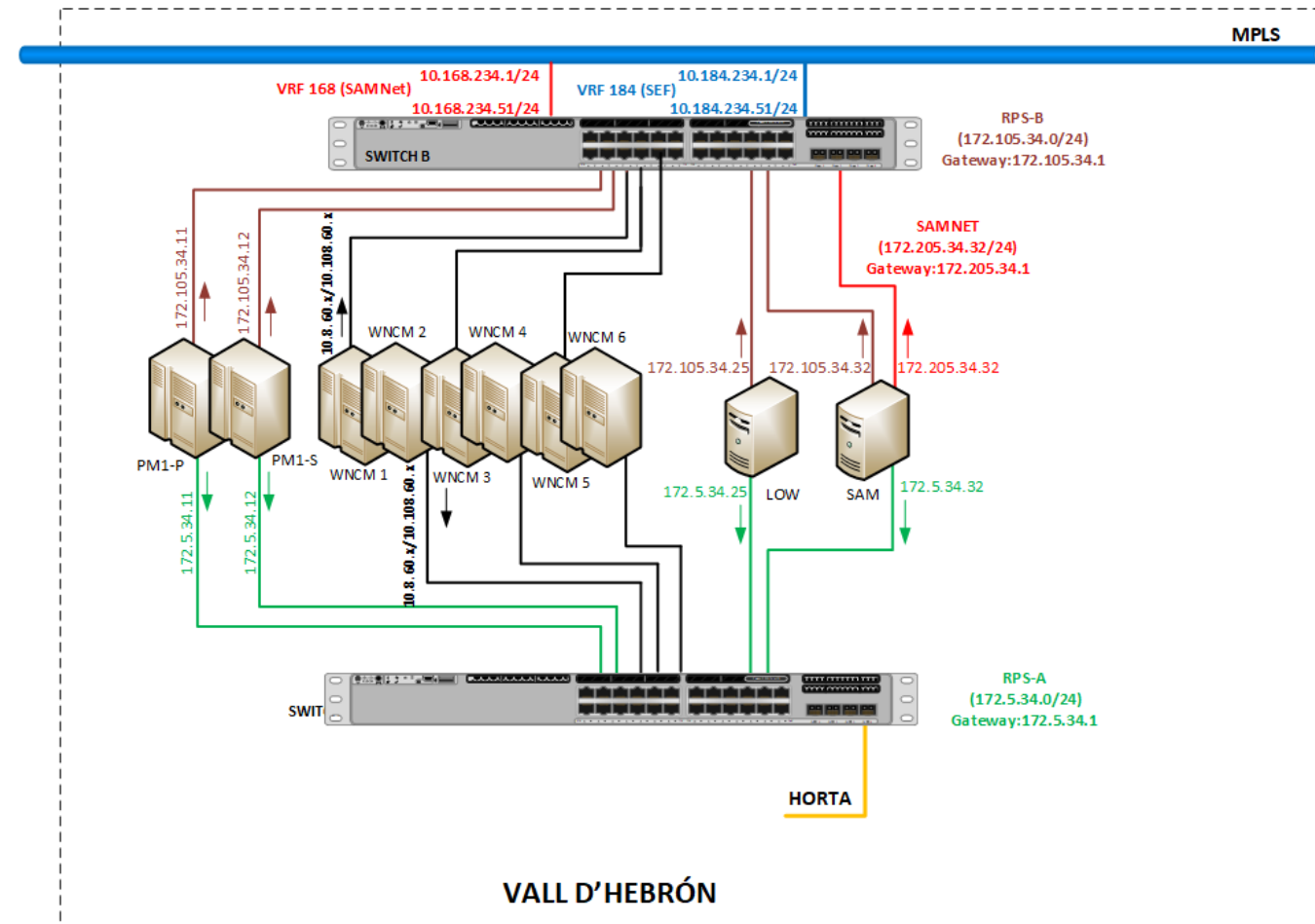
Figura 7 Futura xarxa local de comunicacions de l'enclavament de Vall d'Hebrón.
