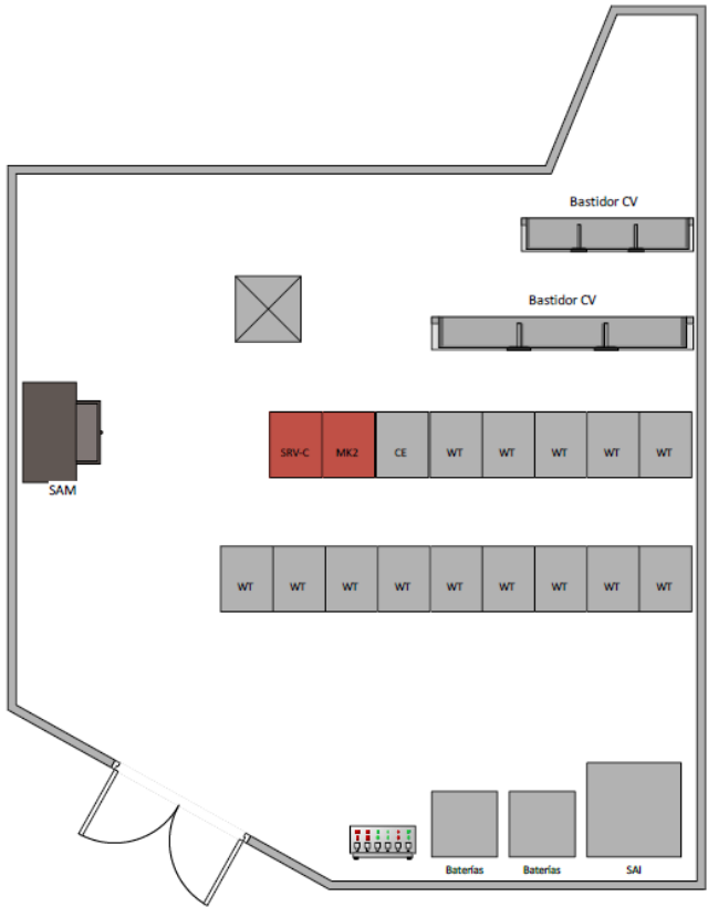
Figura 5 Distribució d'equips proposada per a l'enclavament de Vall d'Hebrón.
