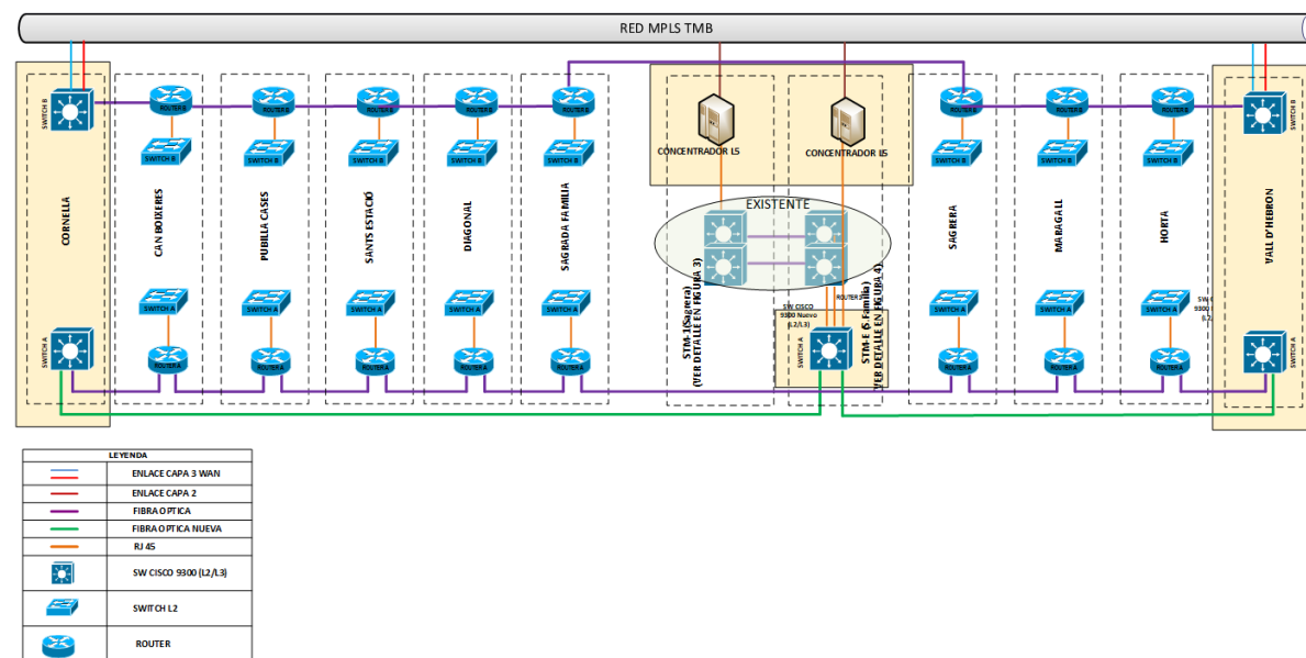
Figura 6. Futura xarxa local de comunicacions de l'enclavament de Vall d'Hebron.
