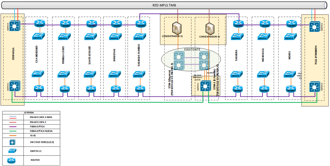
Figura 6 Futura xarxa local de comunicacions de l'enclavament de Vall d'Hebrón.
