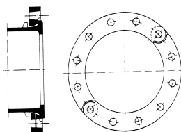
Brida orientable
