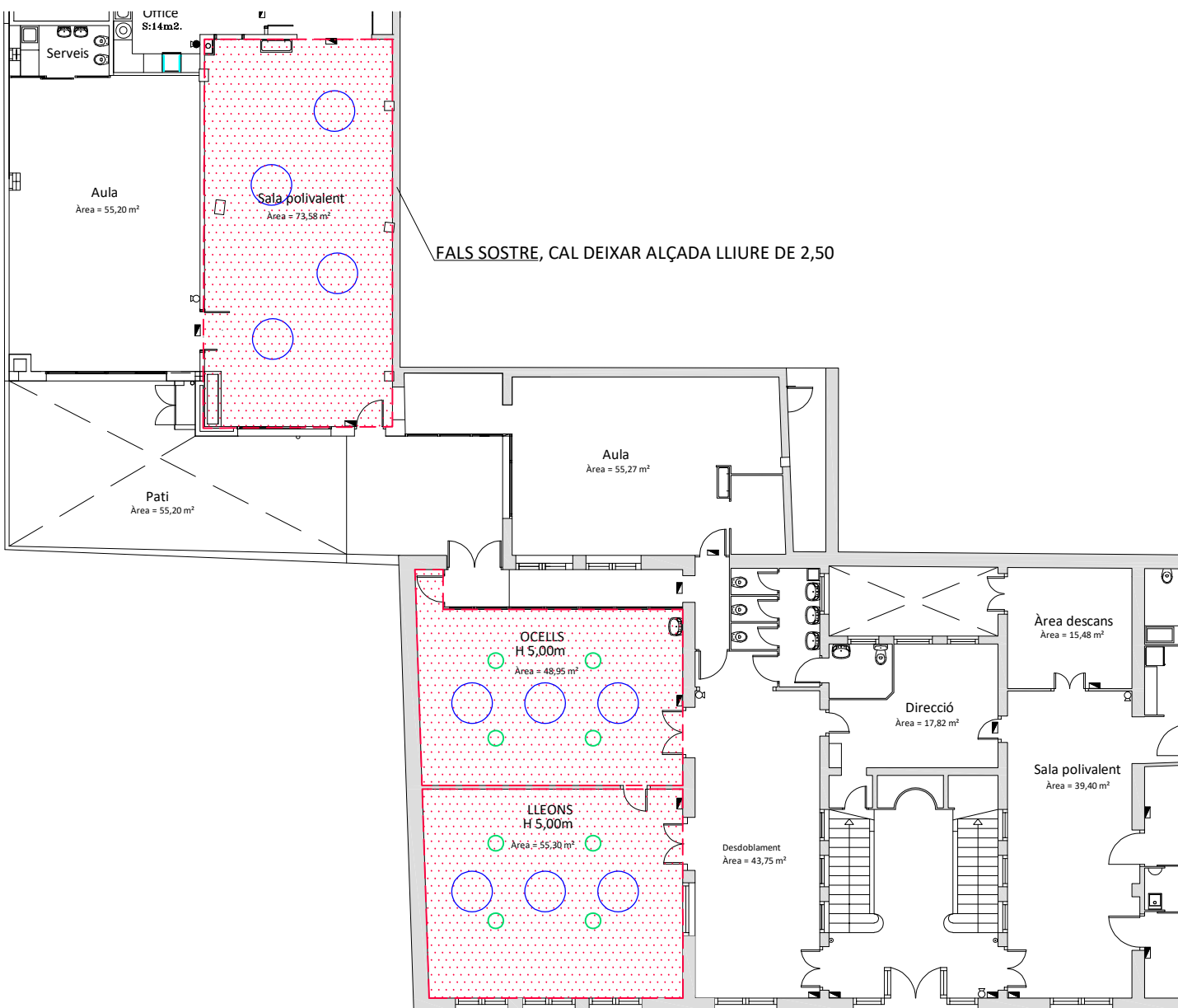
SOSTRES PLANTA BAIXA
