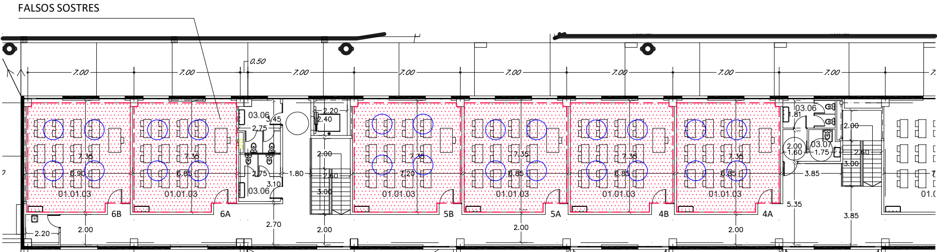
PLANTA SEGONA
