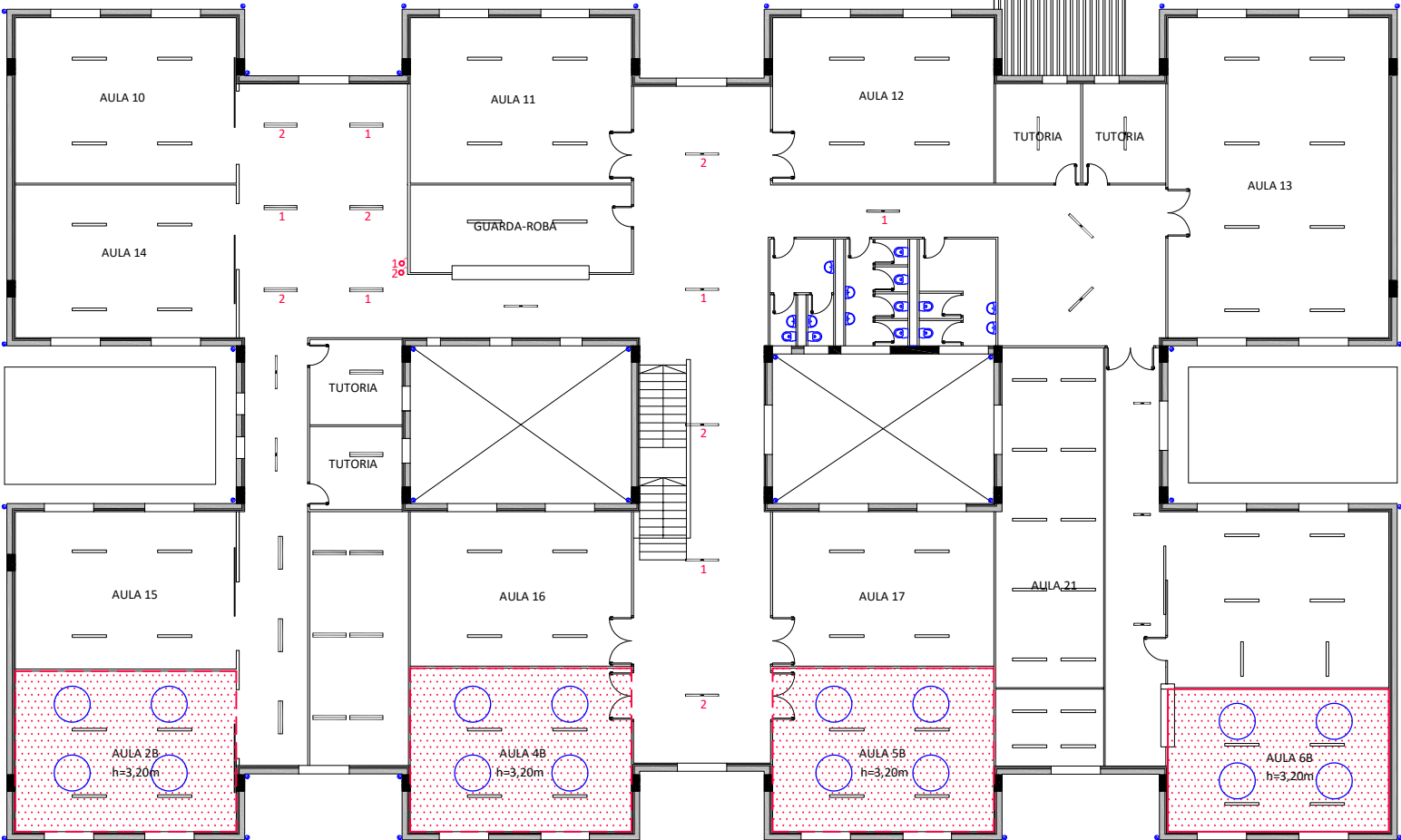
PLANTA PRIMERA
