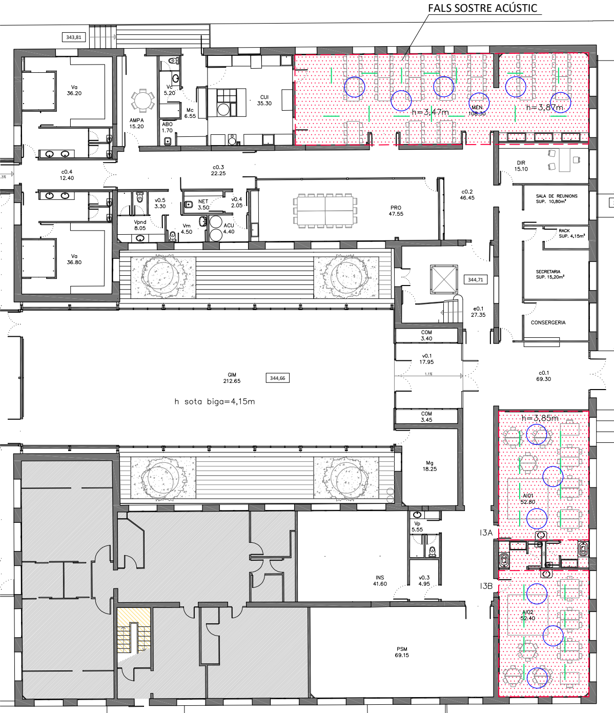
PLANTA BAIXA
