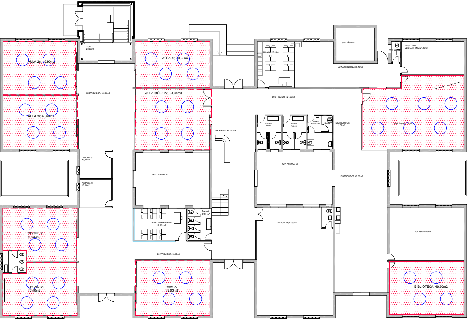
PLANTA BAIXA
