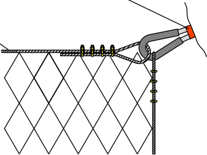
Anclatge de cable GA-7001
