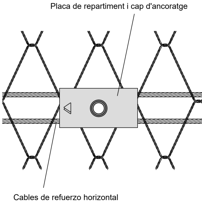
PLACA DE REPARTIMENT
