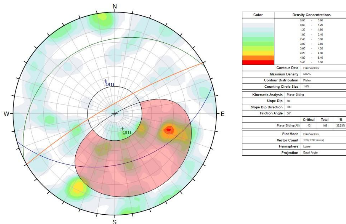
Figura 12. Representació de la cinemàtica i presència de lliscament planar sense límits
