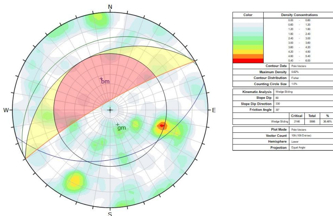
Figura 13. Representació de la cinemàtica i presència de lliscaments a partir de la combinació de plans o el que anomenem falques
