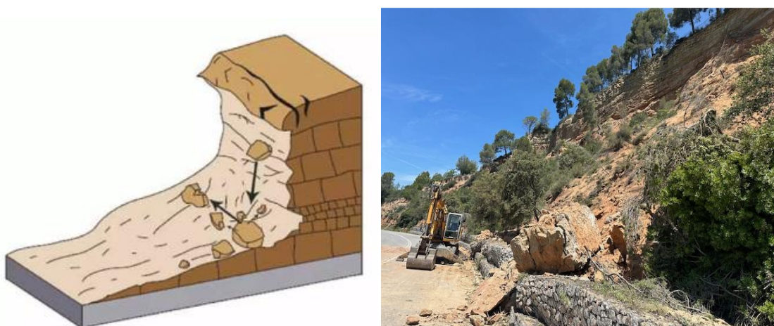
Figura 2. Esquema gràfic de despreniment de roques
