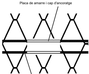
Detall 2 Ancoratge interior i cables de reforç
