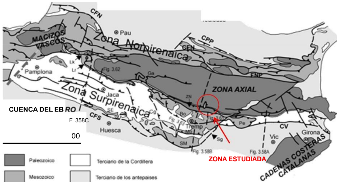
Figura 5. Marc estructural de la serralada dels pirineus.
