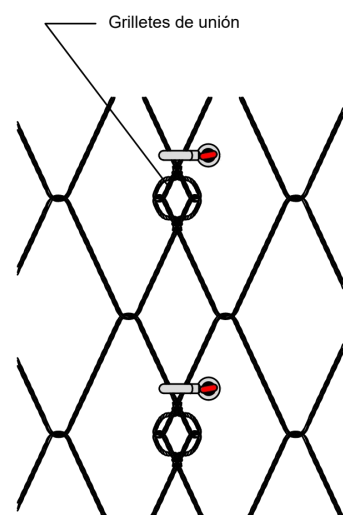
Detalle 1 Unión vertical entre paños
