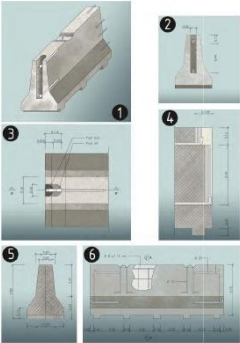
Barrera rígida de formigó (portàtil) 1. Axonòmetrica 2. Alçat transversal 3. Planta detall AA 4. Secció BB 5. Elevation 6. Plan view
