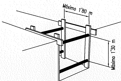
ENTIBACIÓN LIGERA
