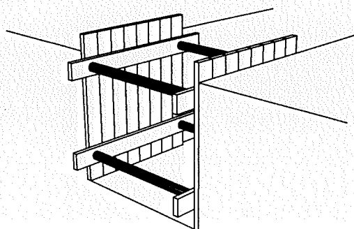
ENTIBACIÓN CUAJADA
