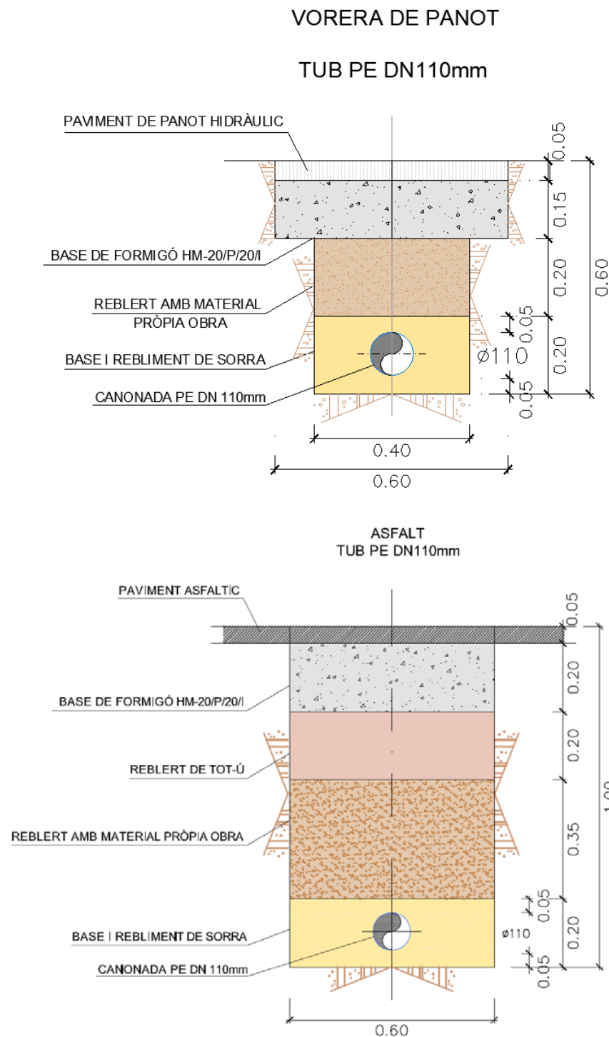
Secció Tipus rasa canonada.
