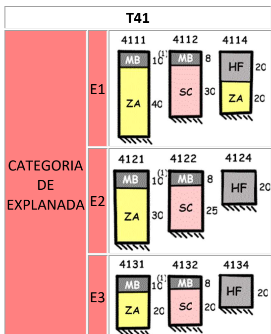
FIGURA 2.2 – CATÁLOGO DE SECCIONES DE FIRME PARA LAS CATEGORÍAS DE TRÁFICO PESADO T3 (T31 y T32) y T4 (T41 y T42), EN FUNCIÓN DE LA CATEGORÍA DE EXPLANADA.
