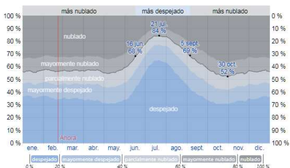
Categoria de nuvolositat
