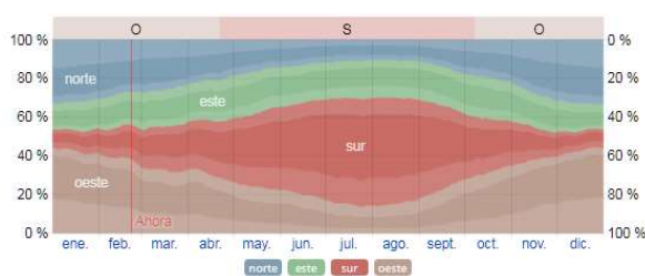
Direcció dels vents superiors a 1.6 km/h.
