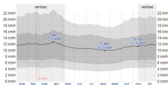
Velocitat mitjana del vent
