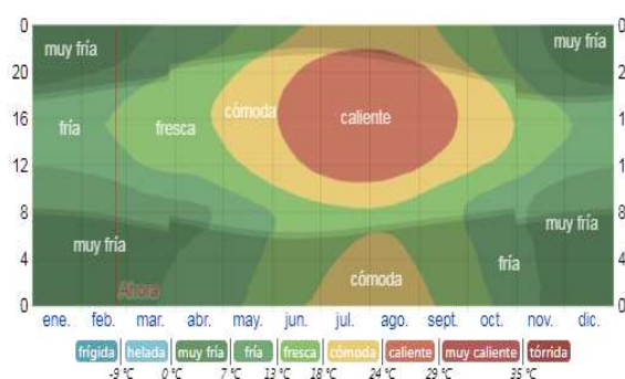
Temperatures mitjanes per hora
