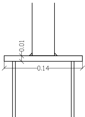
Detall base amb pletina de fixació E:1:10
