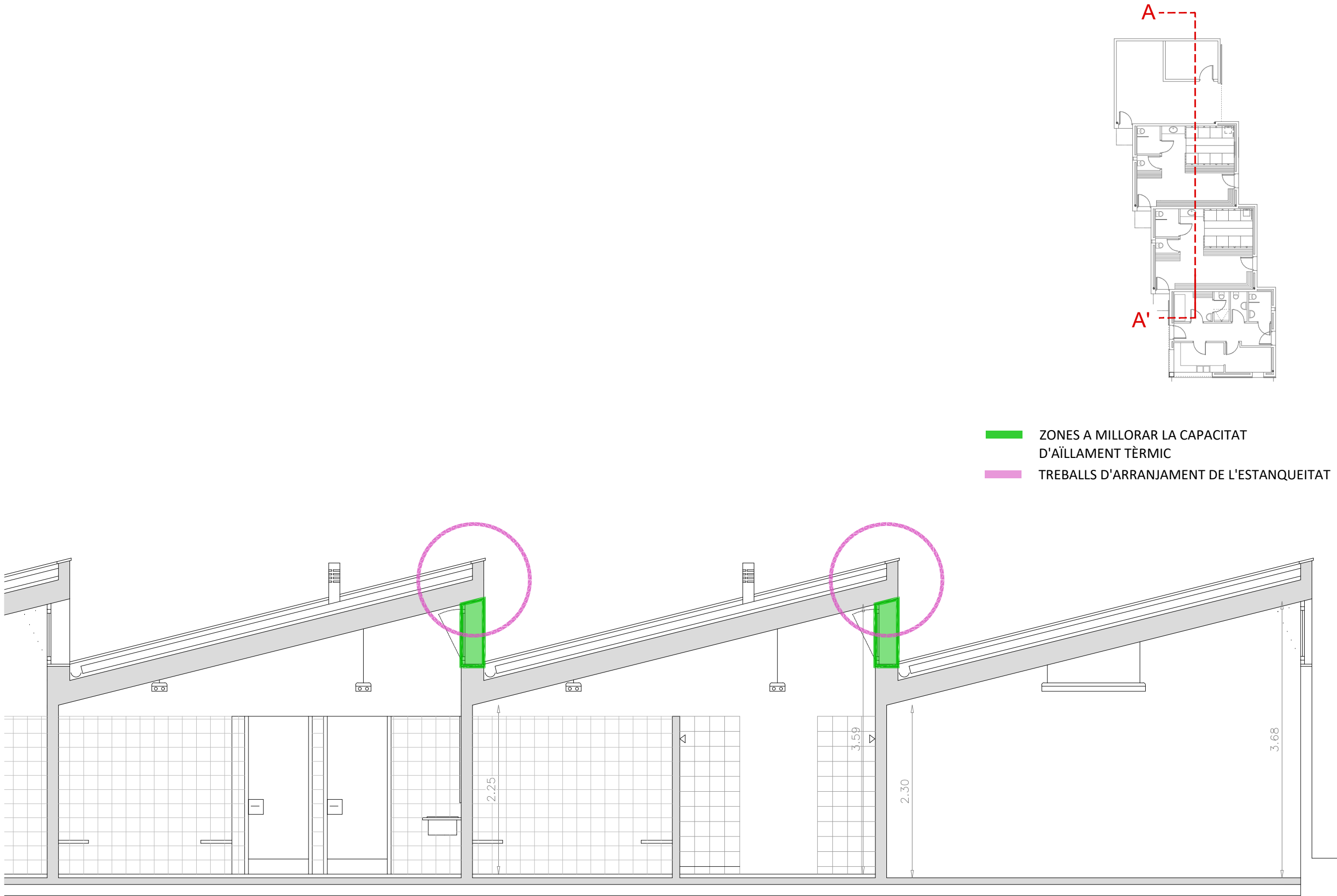
SECCIÓ A-A'
