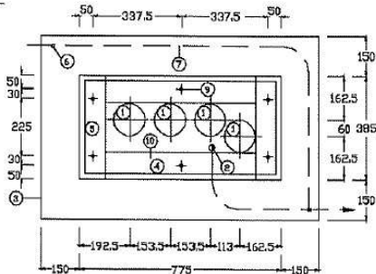
Figura 4: Esquema basament armari Tipus 1
