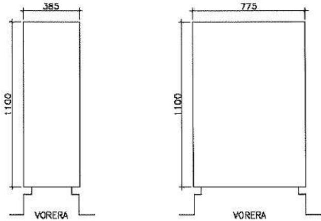
Figura 1 : Armari d'intempèrie TIPUS 1
