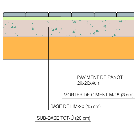
SECCIÓ VORERA AMB PANOT 20x20x4cm ESCALA: 1/20
