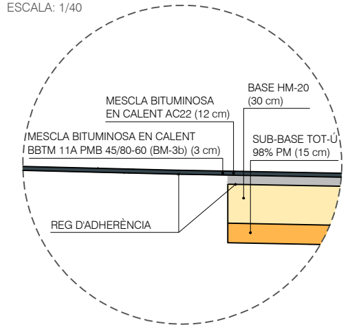
DETALL A ESCALA: 1/40
