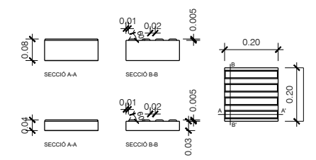
PAVIMENT PODOTÀCTIL ESCALA: 1/20
