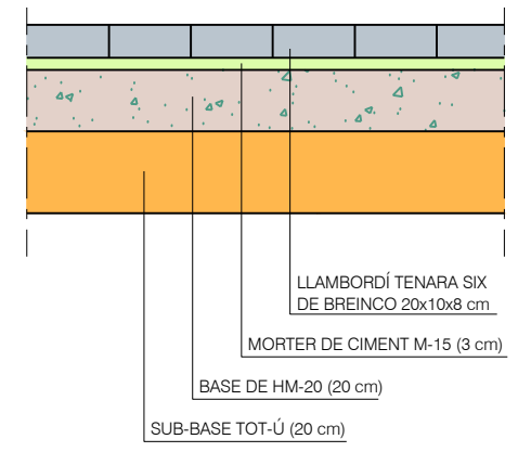
DETALL PAVIMENT DE LLAMBORDA TERANA SIX ESCALA: 1/20
