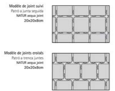
DETALL PAVIMENT DRENANT ESCALA: 1/20
