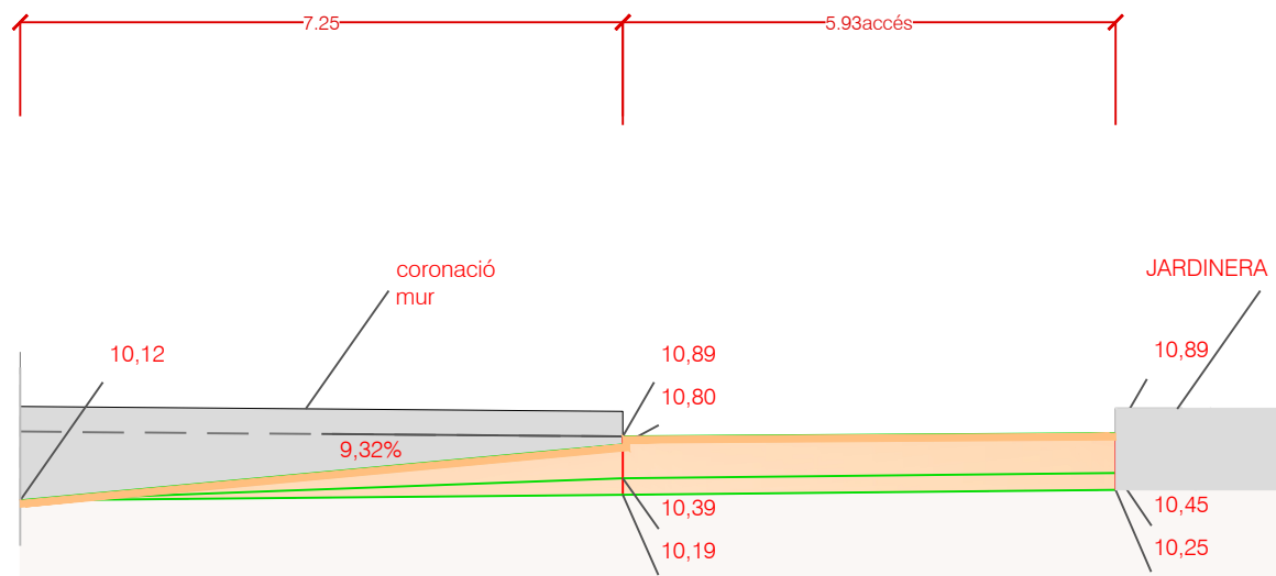
SECCIÓ C-C' ESCALA 1/100
