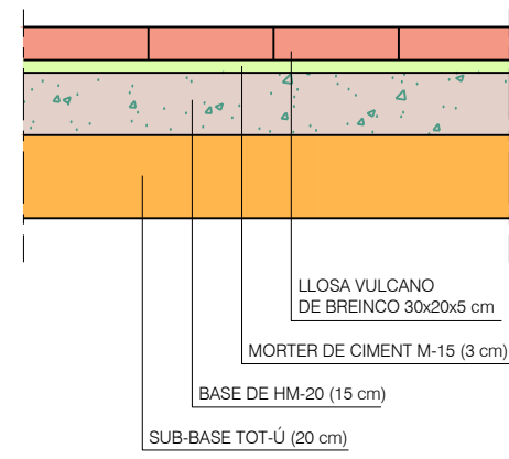
DETALL PAVIMENT LLOSA VULCANO ESCALA: 1/20
