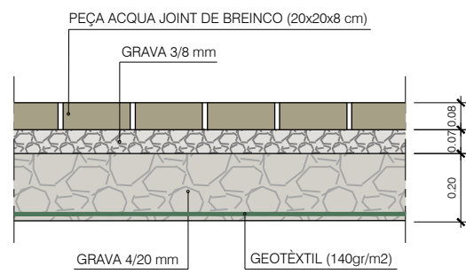
DETALL PAVIMENT DRENANT ESCALA: 1/20
