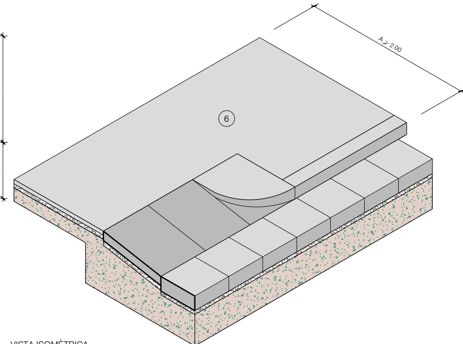
VISTA ISOMÈTRICA
