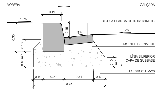
DETALL VORADA TIPUS T-5 AMB RIGOLA DE 0.30x0.30x0.08 ESCALA 1/10
