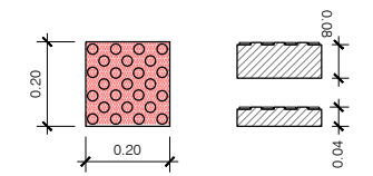
PANOT DE BOTONS ESCALA: 1/20
