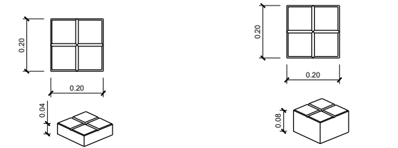
PANOT 4 PASTILLES (PAS VEHICLES) 20x20x8cm ESCALA: 1/20
