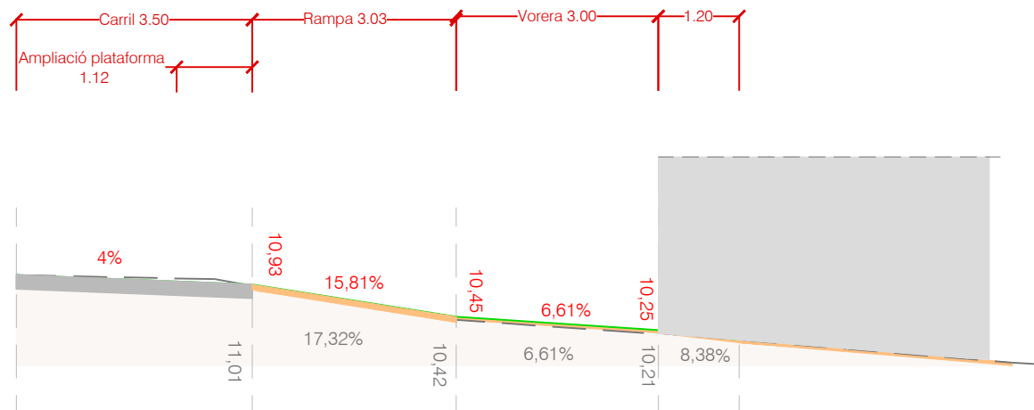
SECCIÓ B-B' ESCALA 1/100
