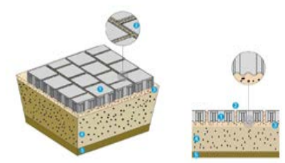
INSTAL·LACIÓ ACQUA JOINT
