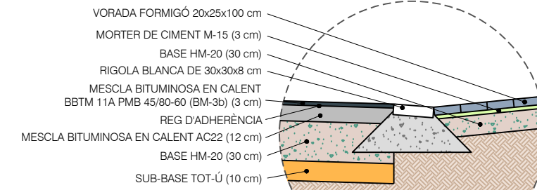
DETALL S3.1 ESCALA: 1/40
