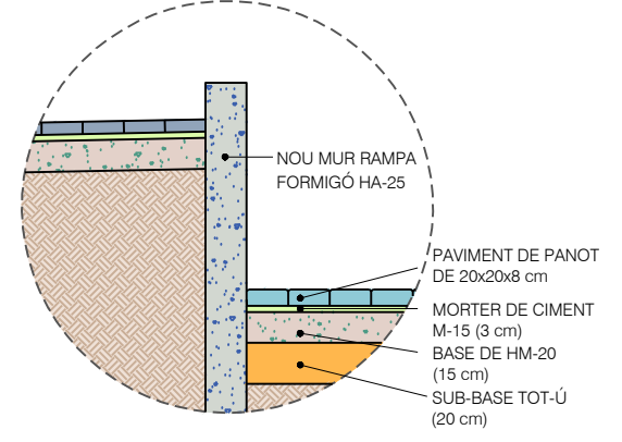
DETALL S3.2 ESCALA: 1/40
