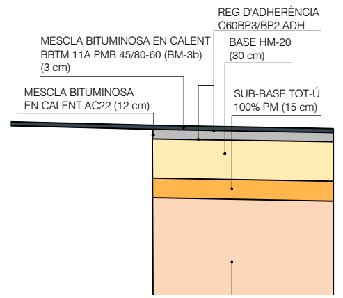
DETALL FERM AMPLIACIÓ CARRIL ESCALA: 1/40
