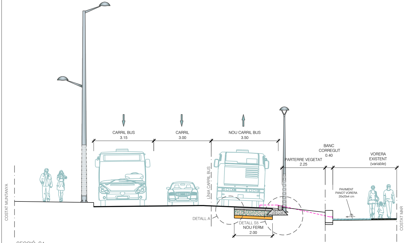
SECCIÓ S4 ESCALA: 1/100
