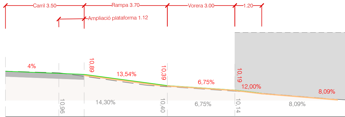
SECCIÓ A-A' ESCALA 1/100
