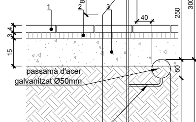
DETALL PAVIMENT DE MICROAGLOMERAT Esc.: 1/10 (cotes en cm)
