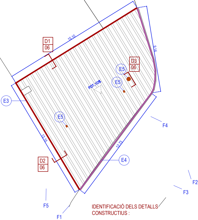
LLAR D'INFANTS ARNAU MIR PLANTA COBERTA E 1/200
