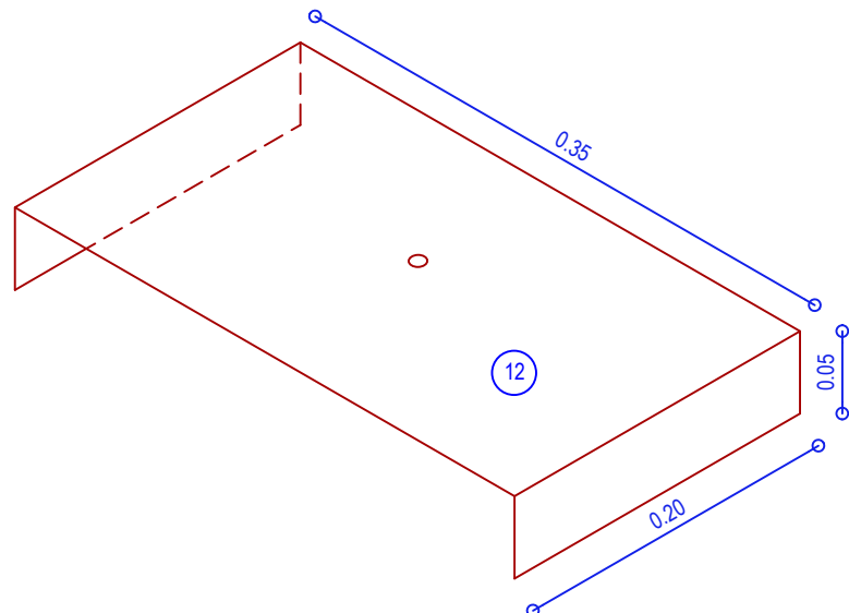
DETALL 9. FIXACIÓ DE XAPA DEL CAVALLÓ. COL·LOCACIÓ CADA 1,5 m E 1/5
