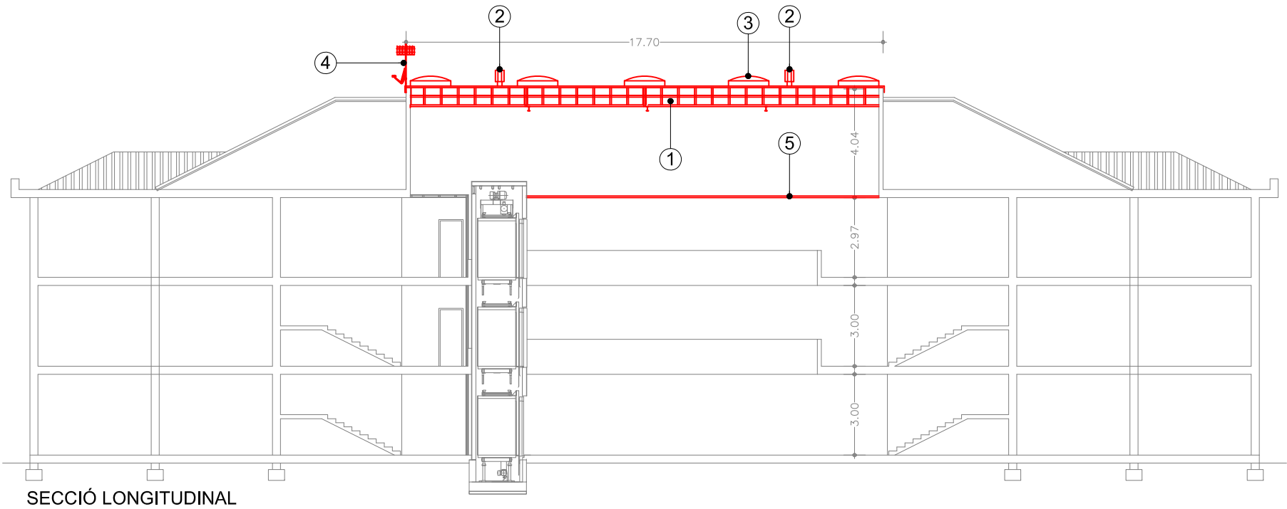
SECCIÓ LONGITUDINAL
