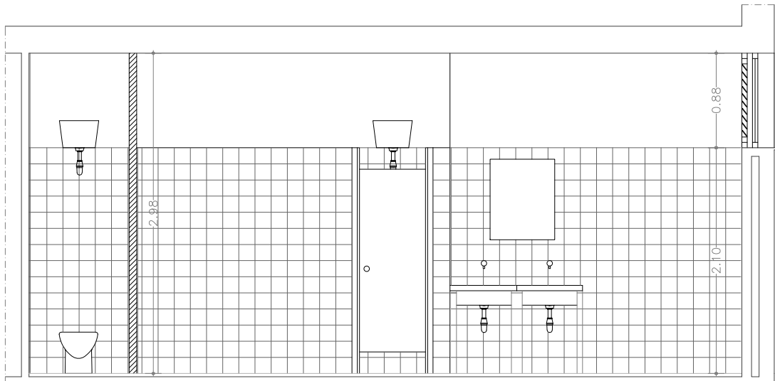
SECCIÓ S1
