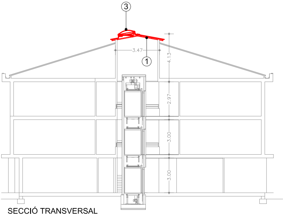
SECCIÓ TRANSVERSAL
