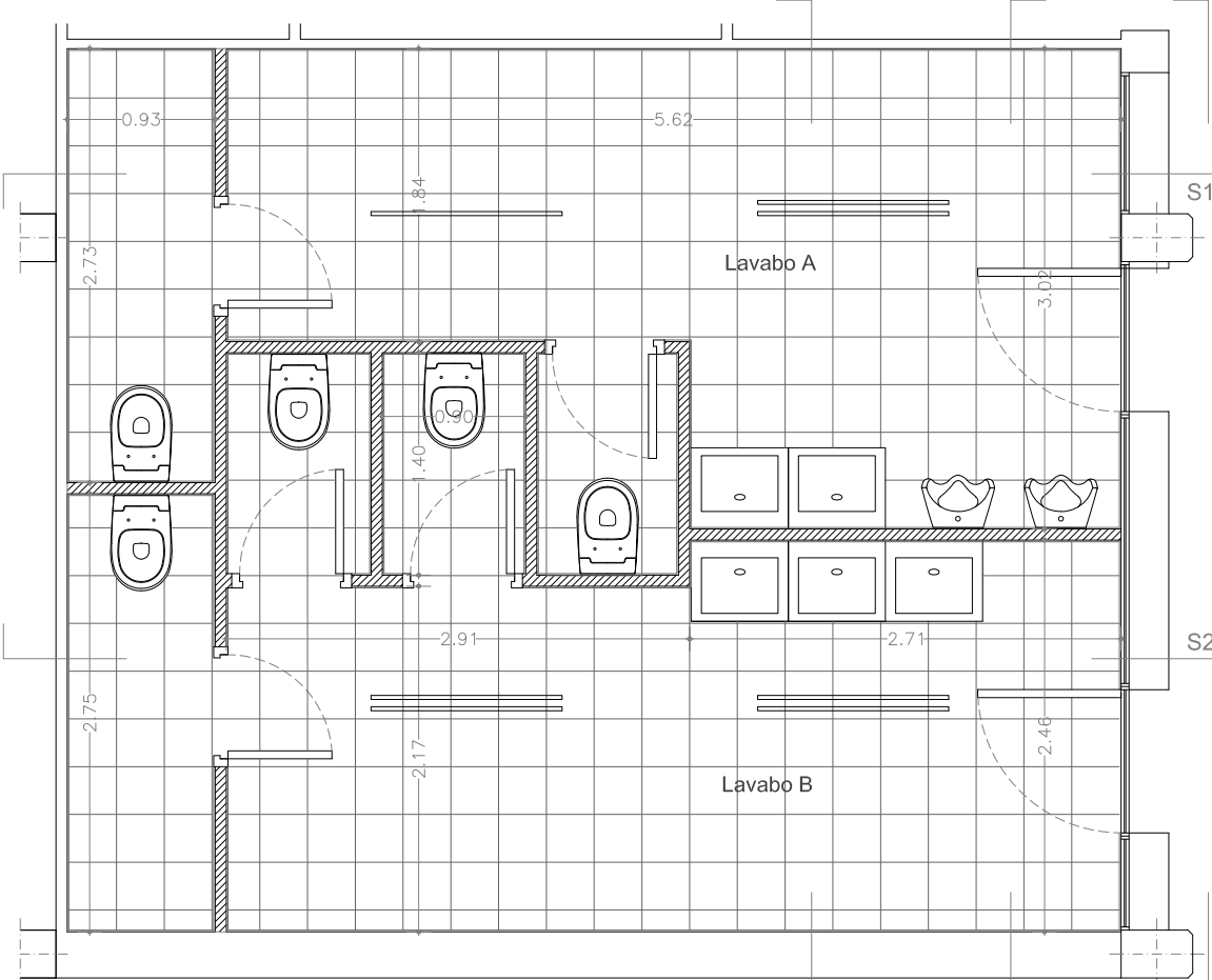
S3
