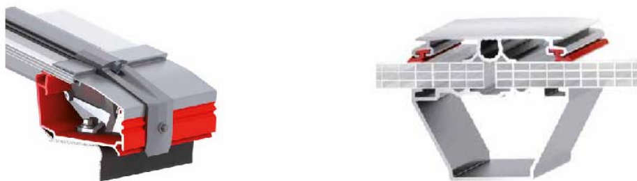
Exemples perfils i envidrament Lluernari tipus B CI-SYSTEM PREFIRE-LAMINUX
