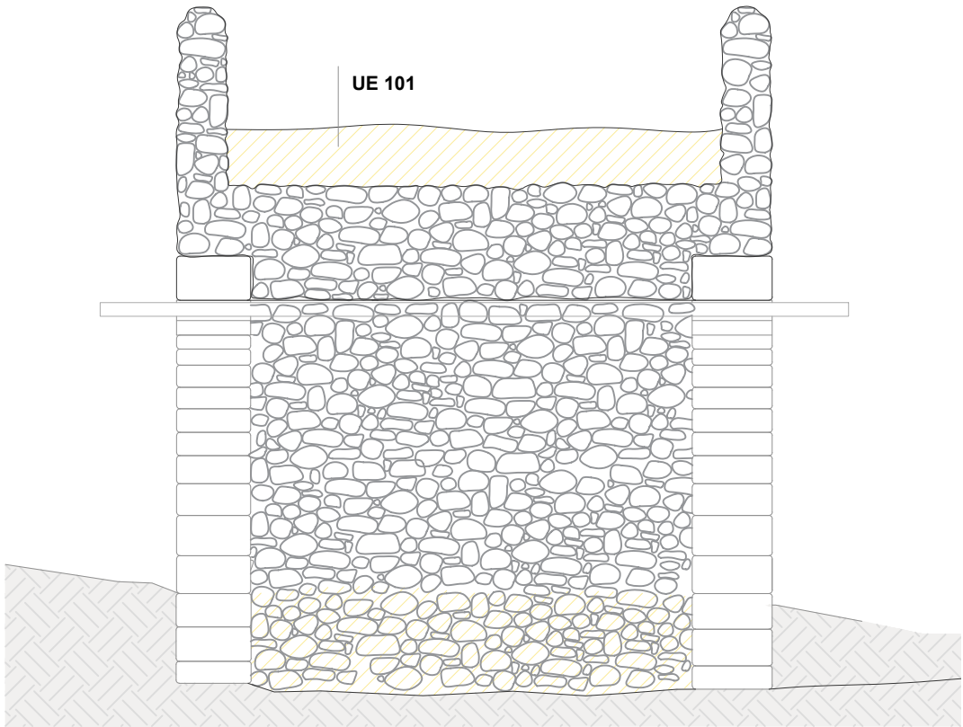
Secció B-B'
