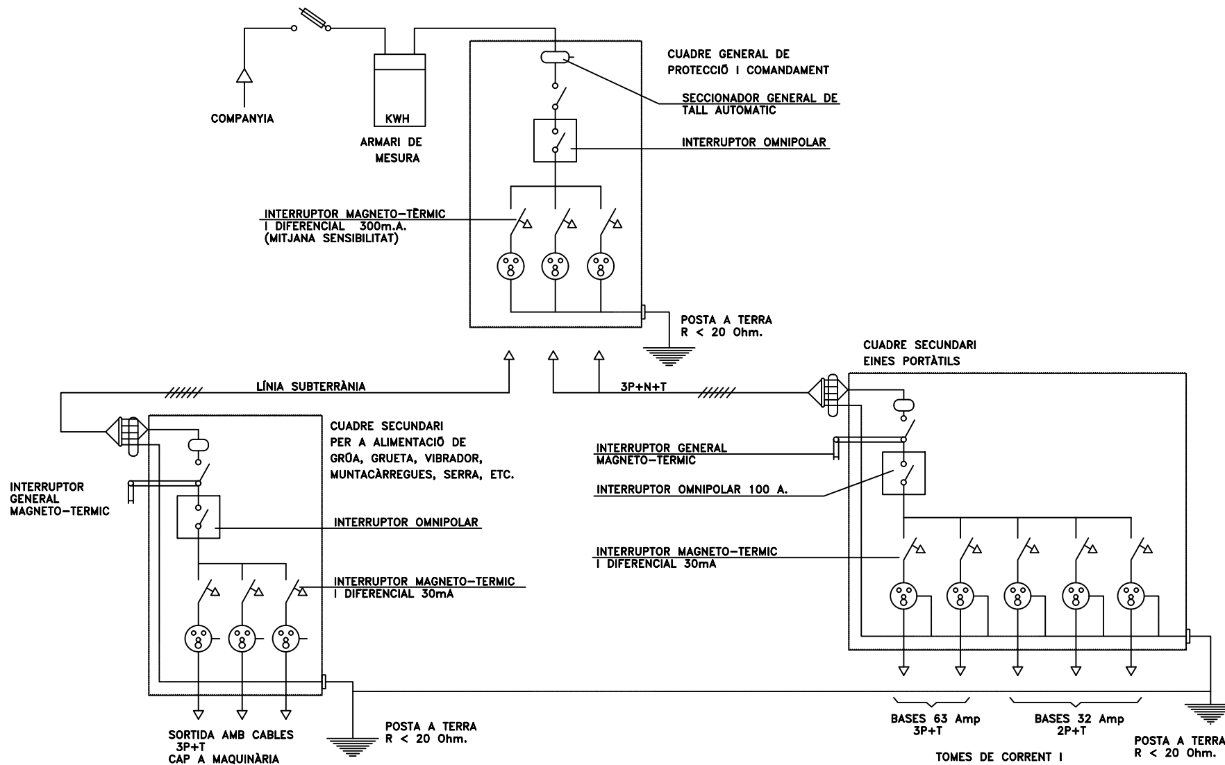
A -EL INTERRUPTOR DIFERENCIAL LIMITA LA INTENSITAT I EL TEMPS, L'DEFECTE.
