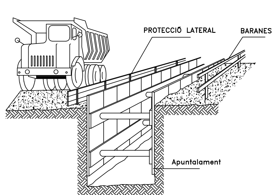
SANEJAMENT HORIZONTAL
