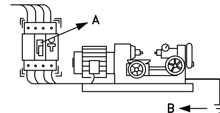
A -EL INTERRUPTOR DIFERENCIAL LIMITA LA INTENSITAT I EL TEMPS, L'DEFECTE.
