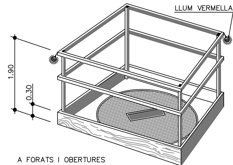
PROTECCIÓ EN RASES
